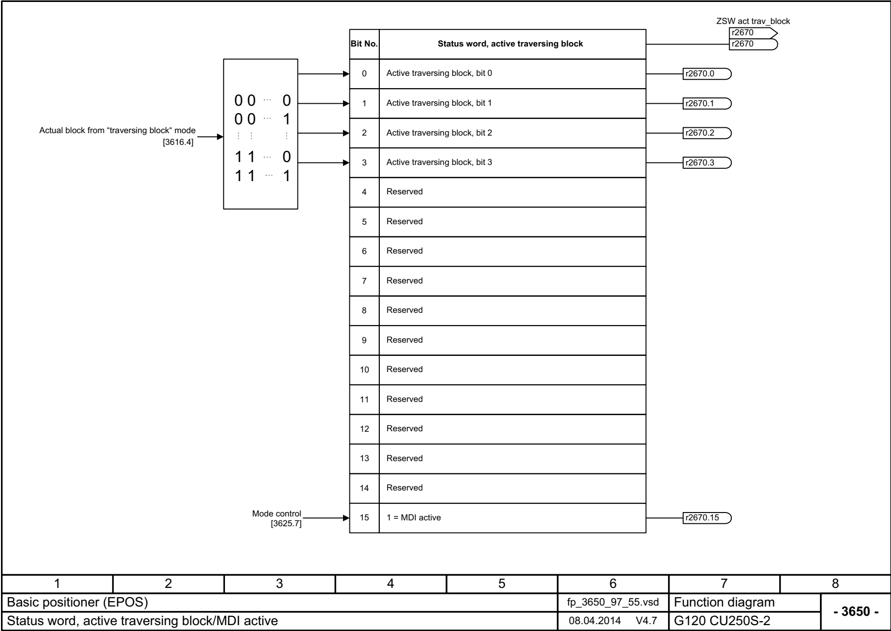
图 3-119 3650 - 有效运行程序段 / 有效 MDI 状态字
