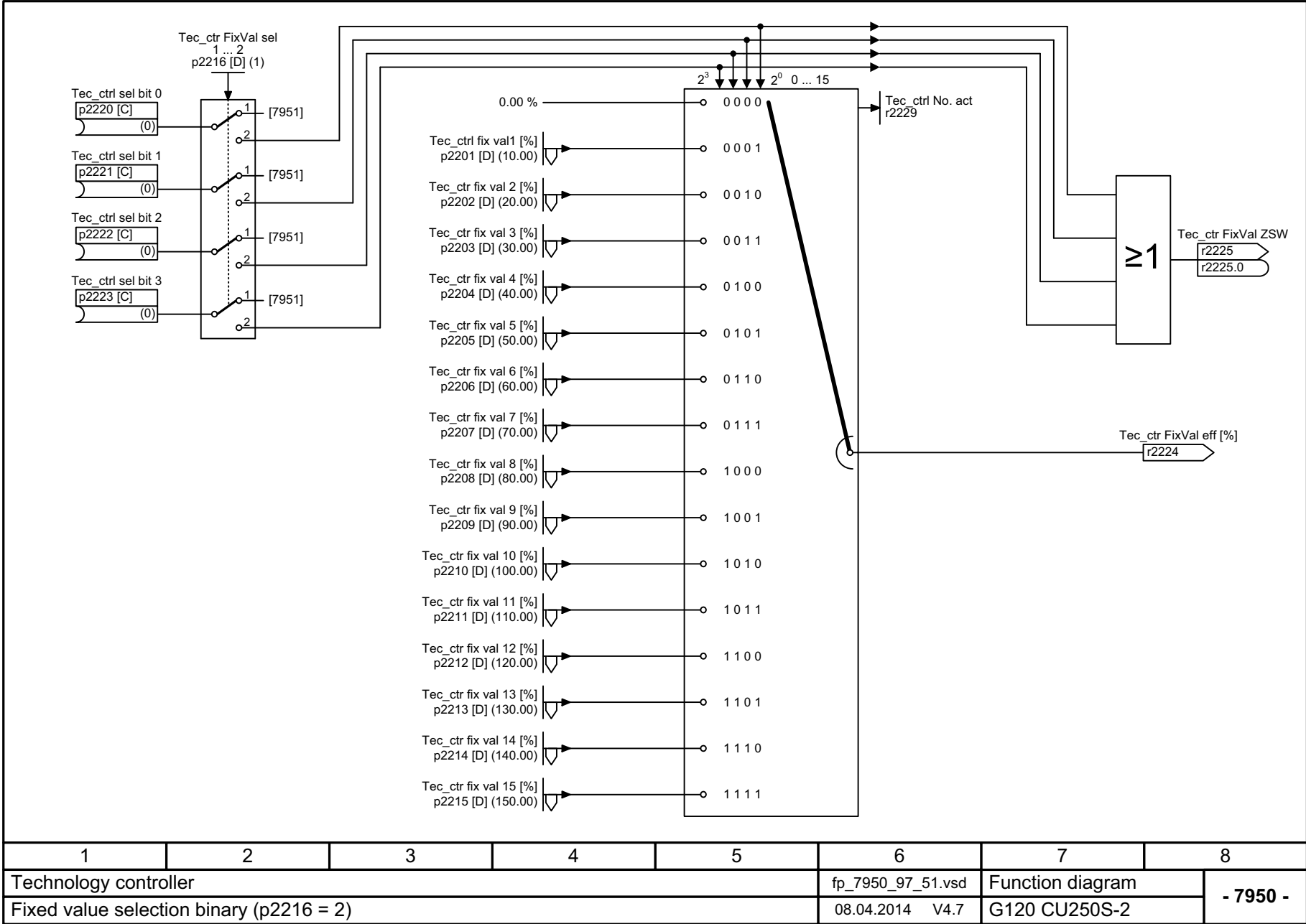
图 3-176 7950 - 固定值, 二进制选择 (p2216 = 2)
