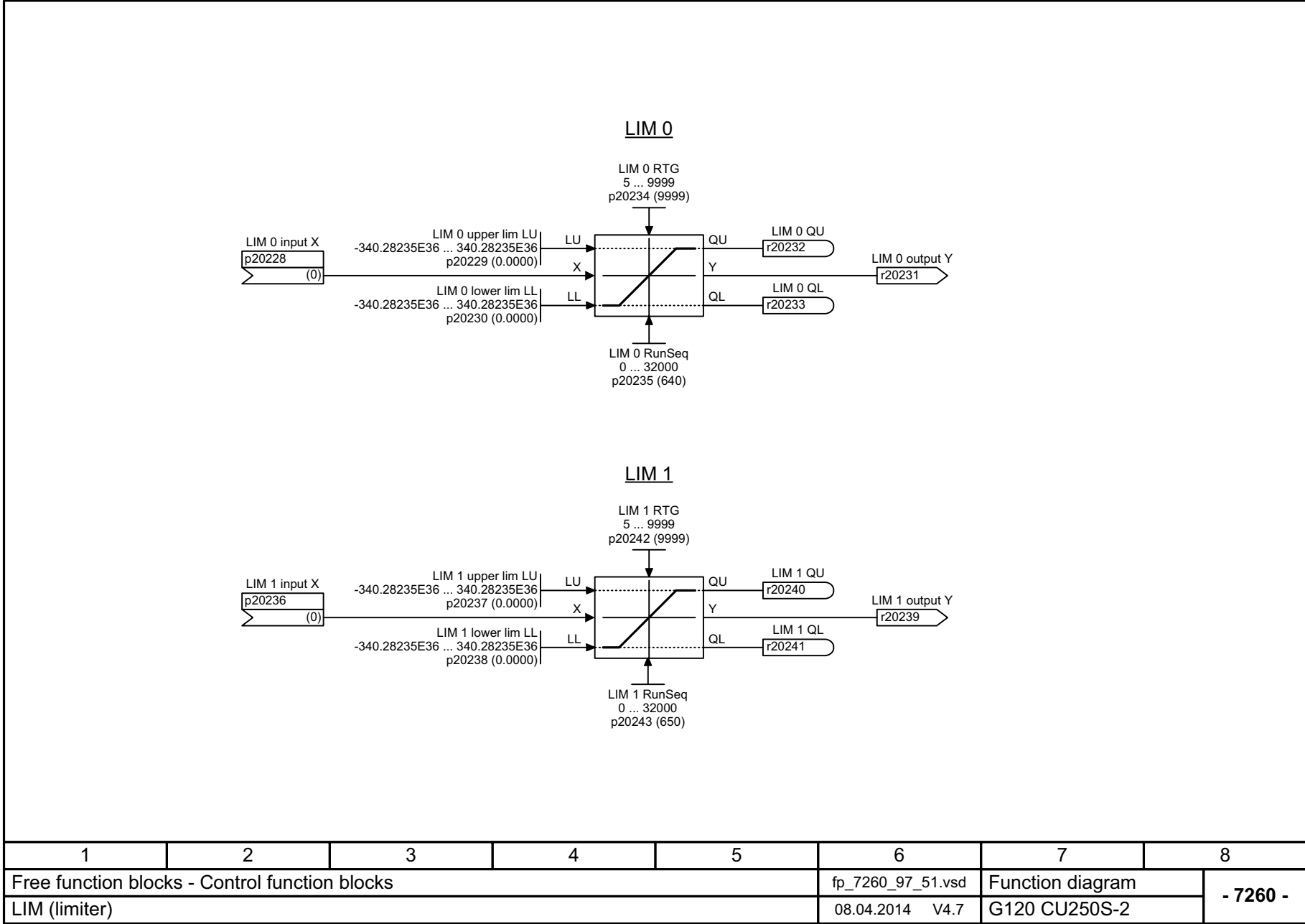
图 3-172 7260 - LIM (限制器)
