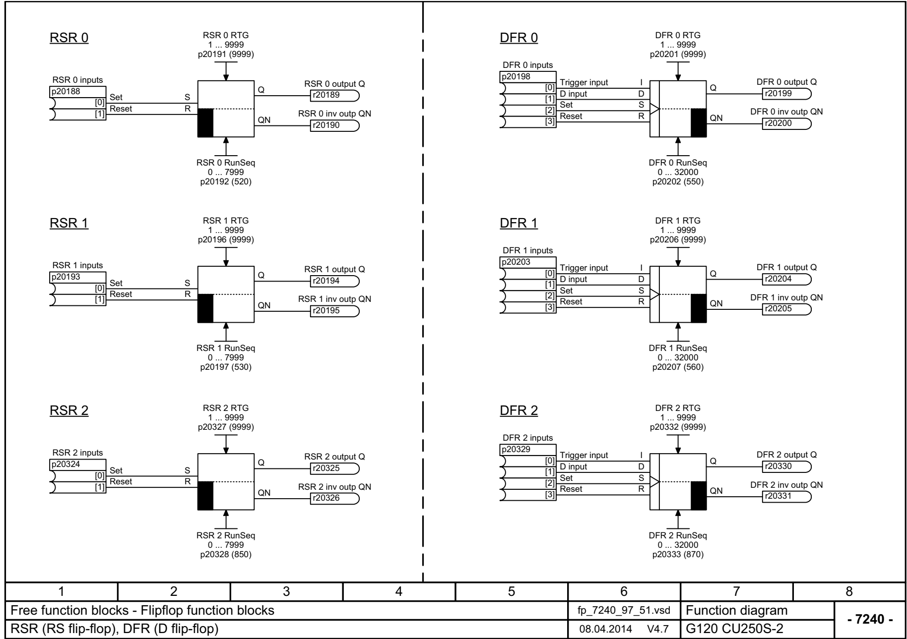
图 3-170 7240 - RSR (R 主导的 RS 触发), DFR (R 主导的 D 触发器)
