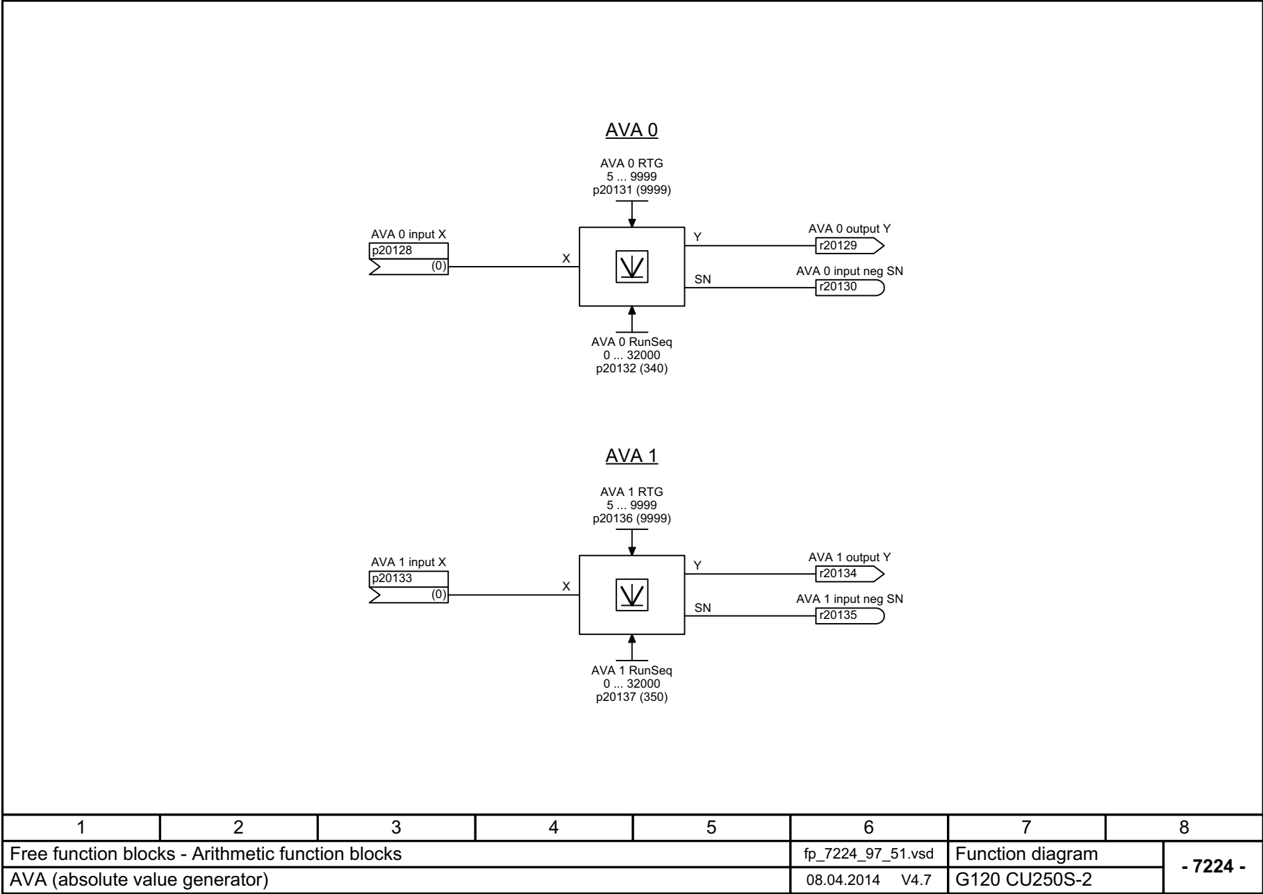
图 3-163 7224 - AVA (绝对值计算器)
