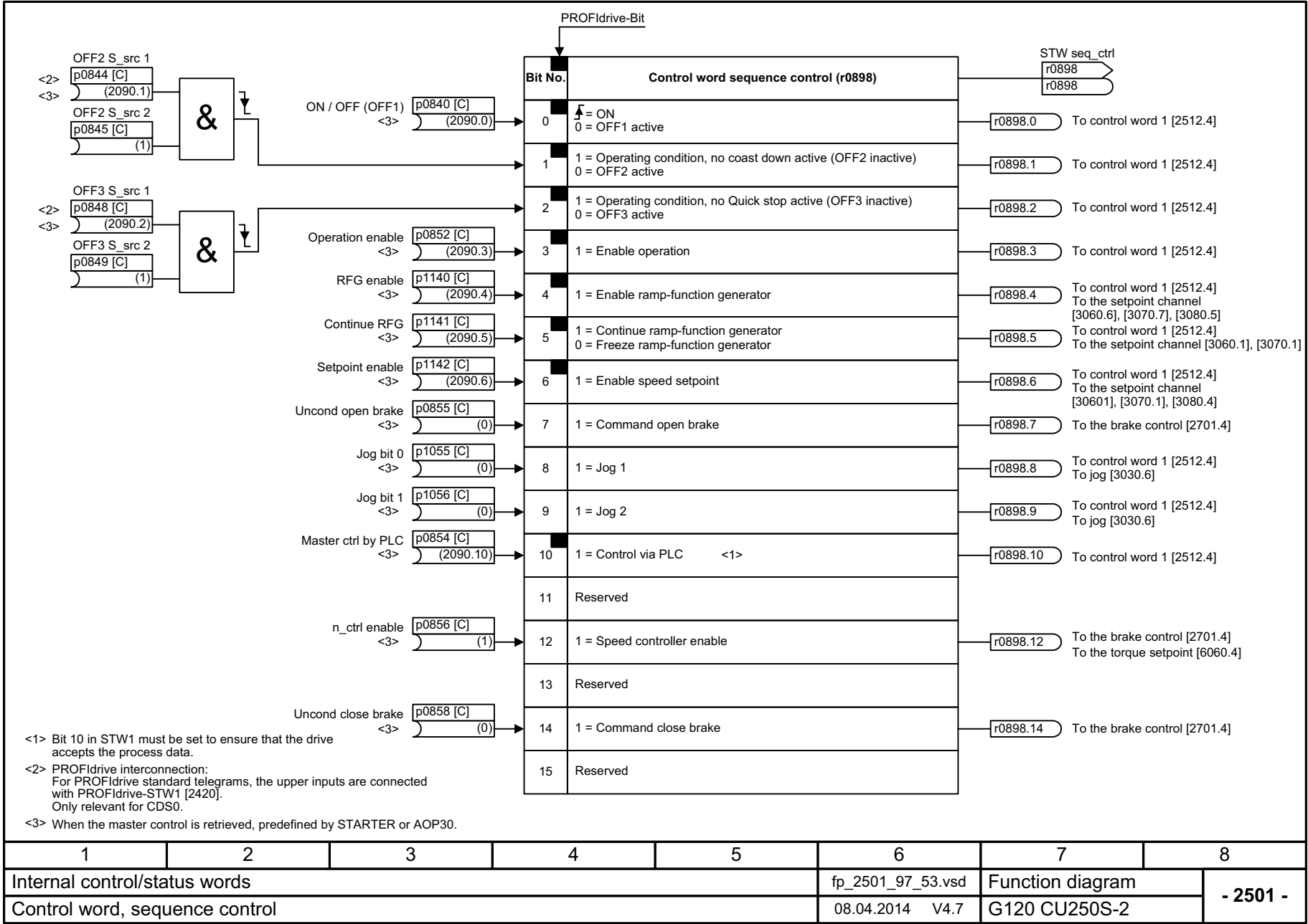
图 3-56 2501 - 顺序控制控制字
