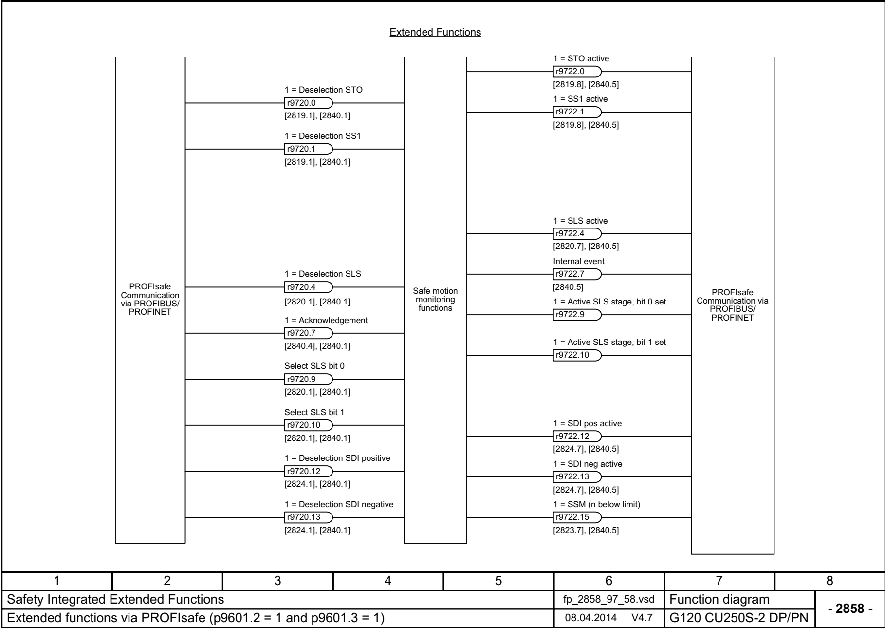
图 3-91 2858 - 扩展功能, 通过 PROFIsafe (9601.2 = 1 和 9601.3 = 1)
