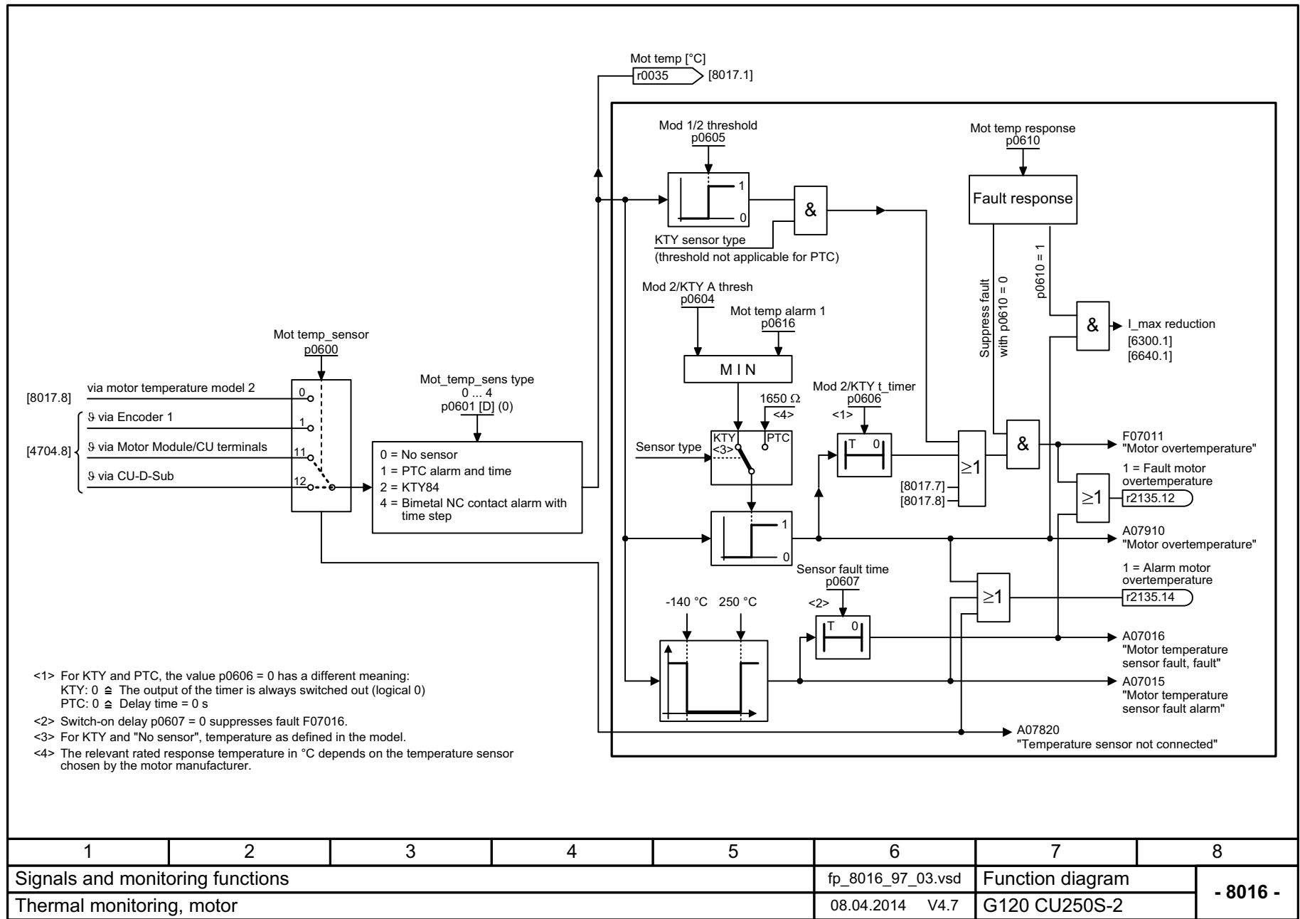
图 3-186 8016 - 电机热负荷监控
