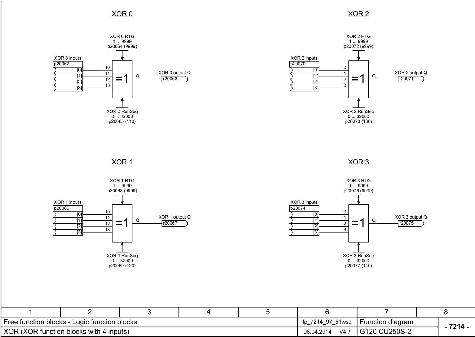
图 3-159 7214 - XOR (有 4 个输入的“异或”功能块)
