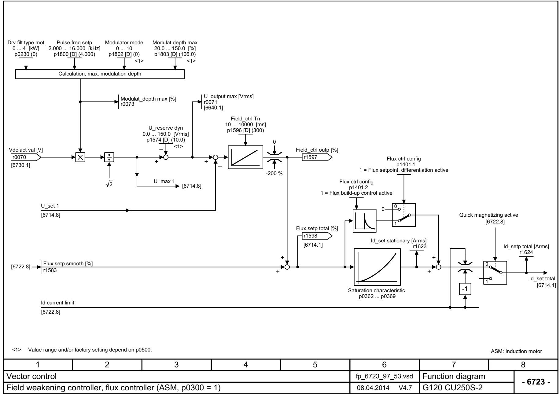
图 3-150 6723 - 去磁调节器, 磁通调节器 (ASM, p0300 = 1)
