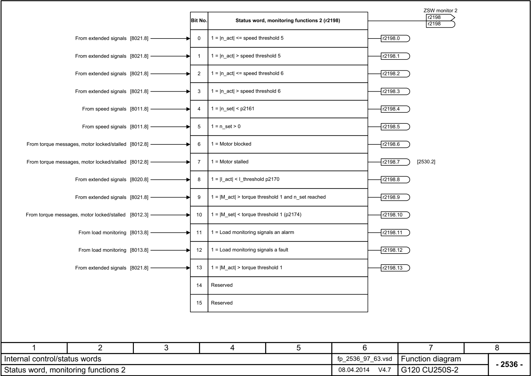
图 3-68 2536 - 监控 2 状态字
