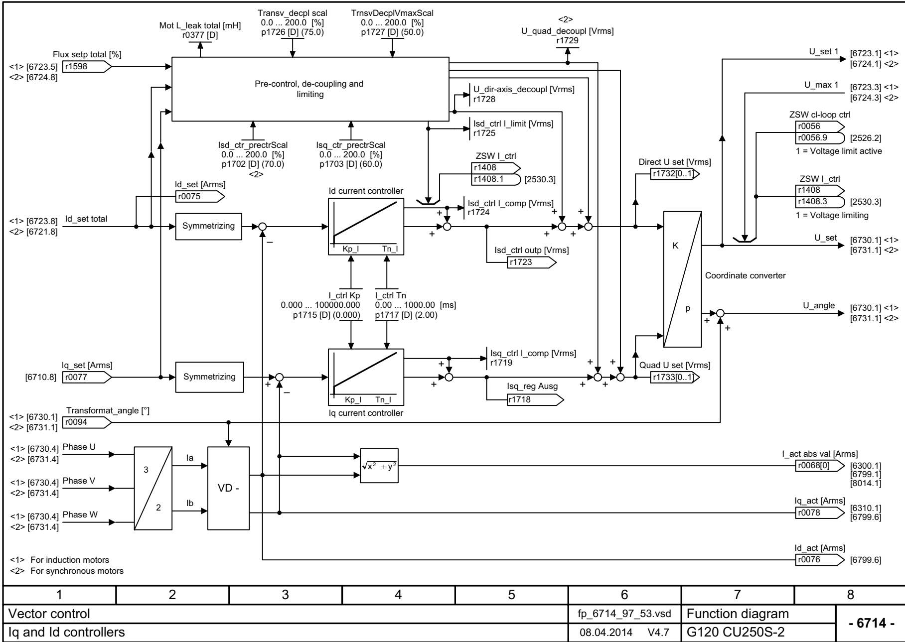
图 3-147 6714 - Iq 控制器和 Id 控制器
