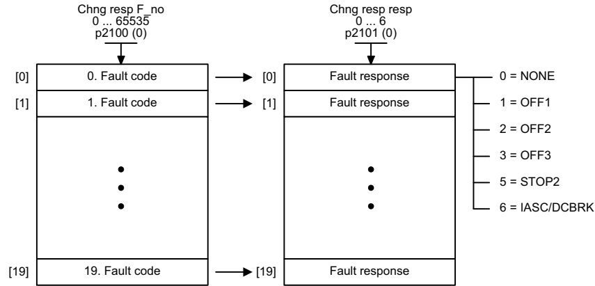
图 3-194 8075 - 故障 / 报警配置
