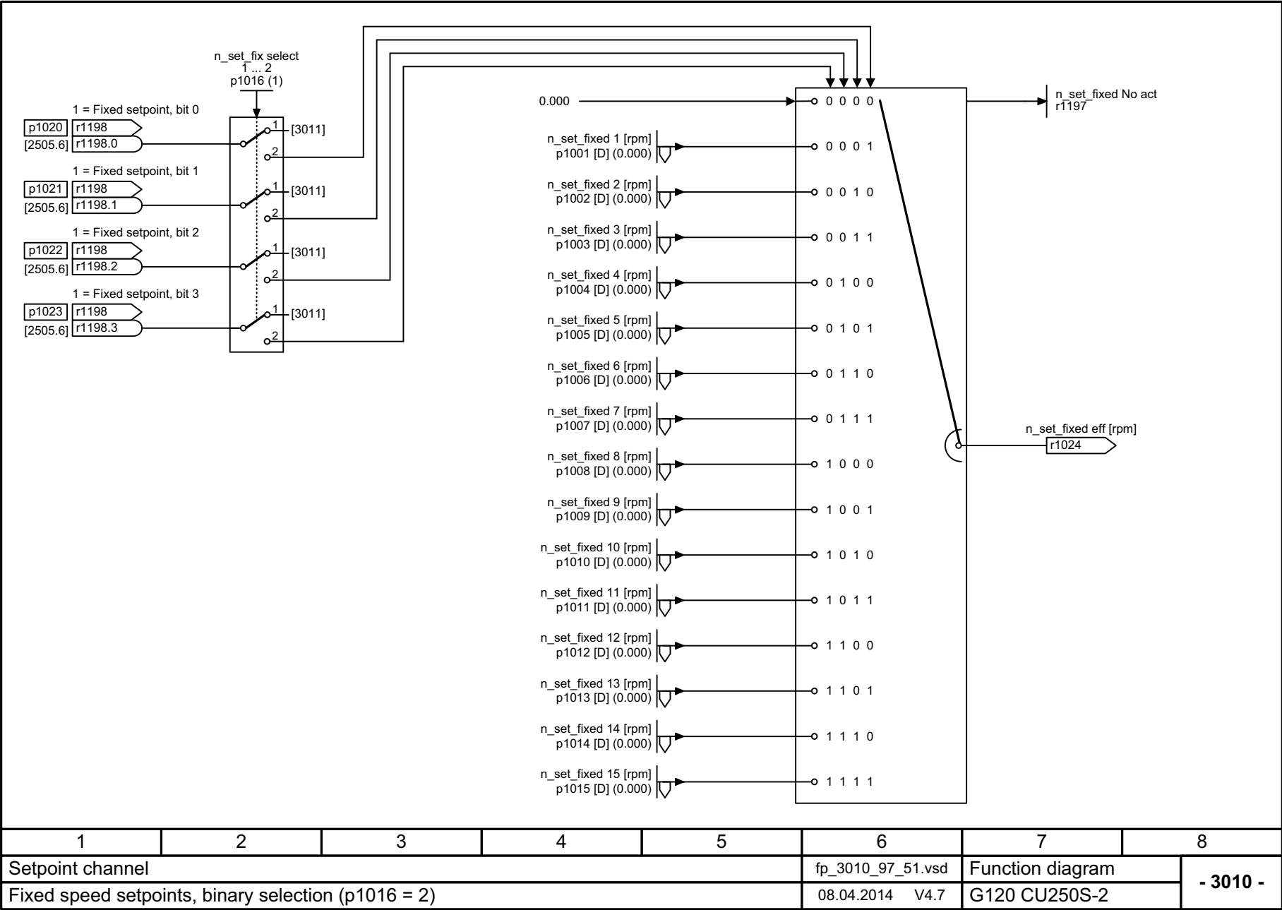
图 3-95 3010 - 转速固定设定值, 二进制选择 (p1016 = 2)
