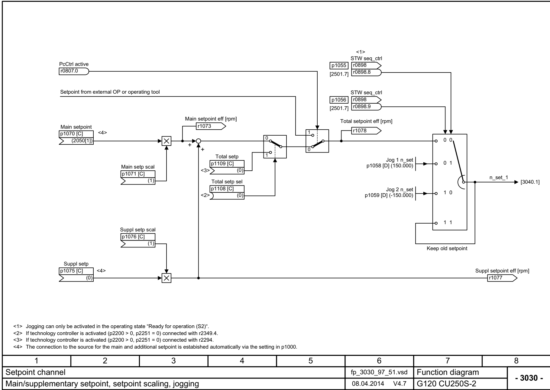
图 3-98 3030 - 主设定值 / 附加设定值, 设定值比例缩放, 点动
