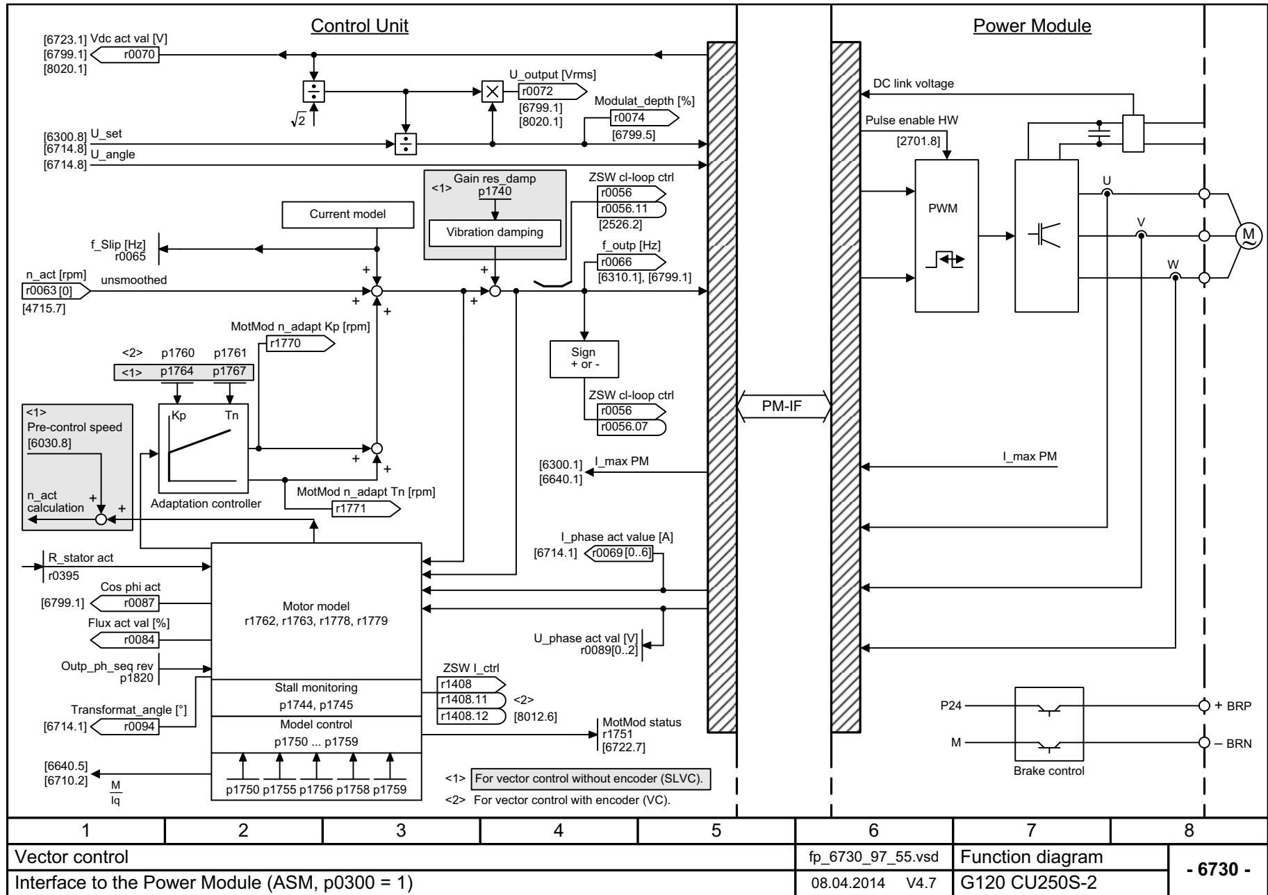
图 3-152 6730 - 和功率模块的接口 (ASM, p0300 = 1)
