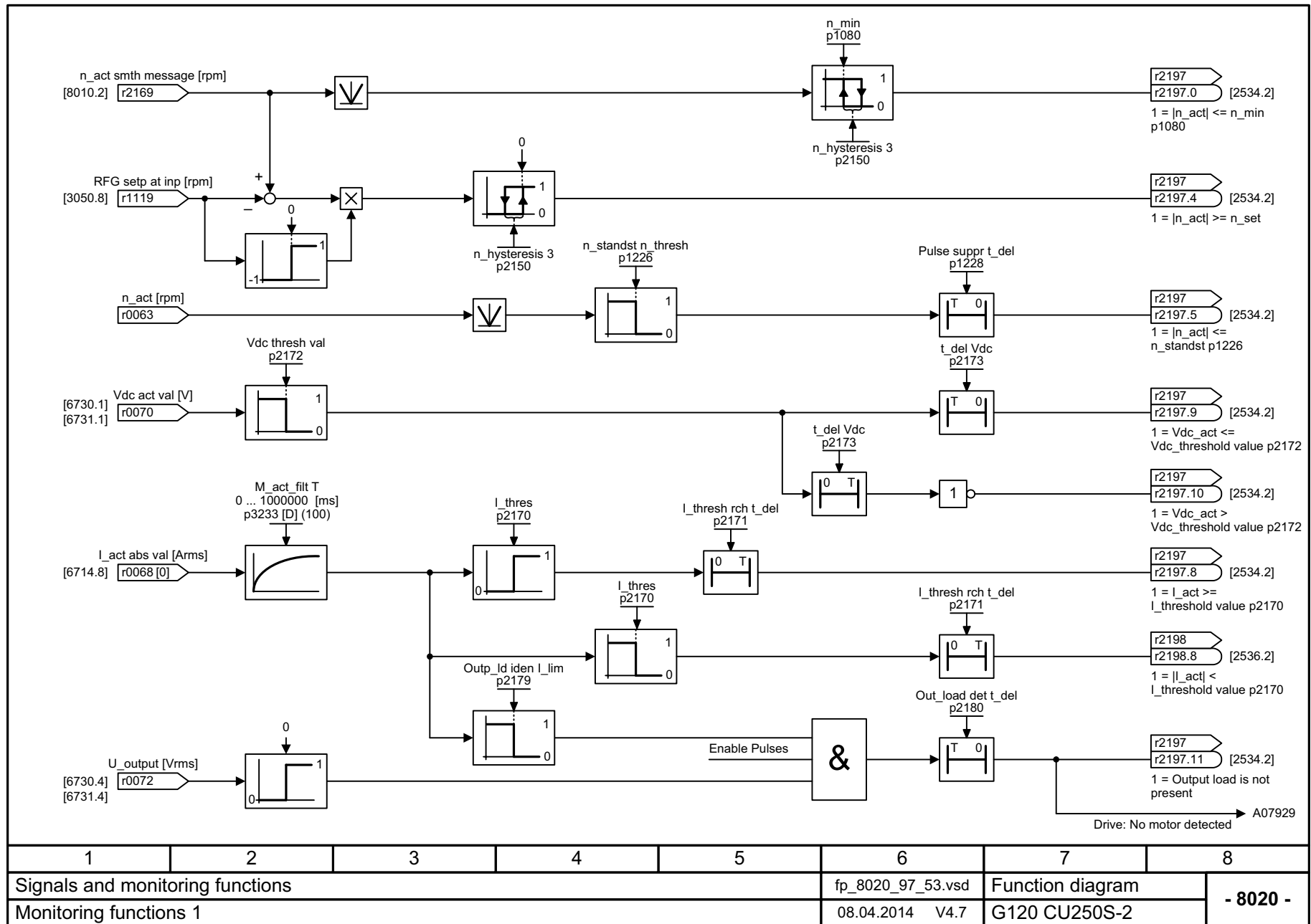
图 3-188 8020 - 监控功能 1
