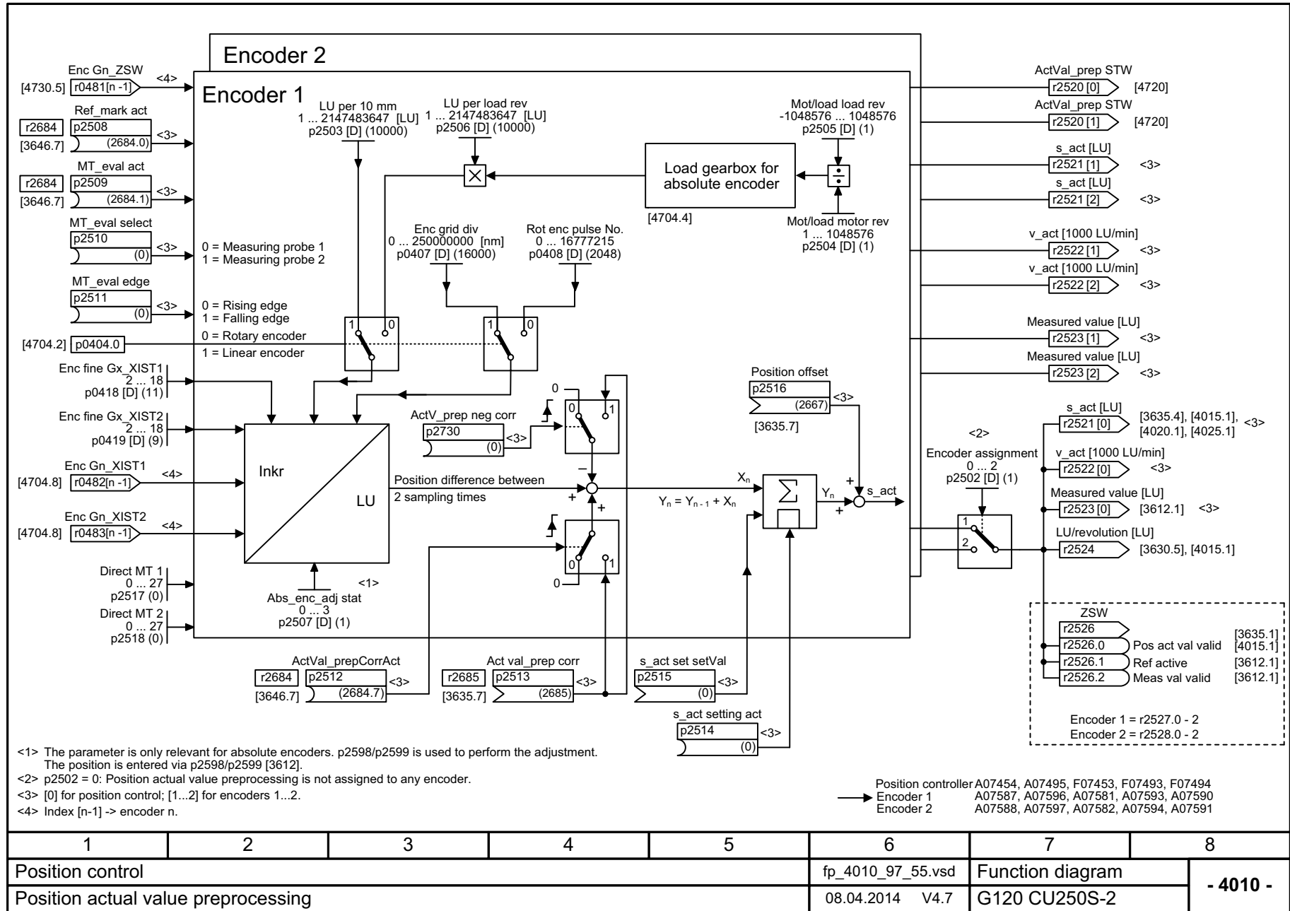
图 3-120 4010 - 位置实际值处理
