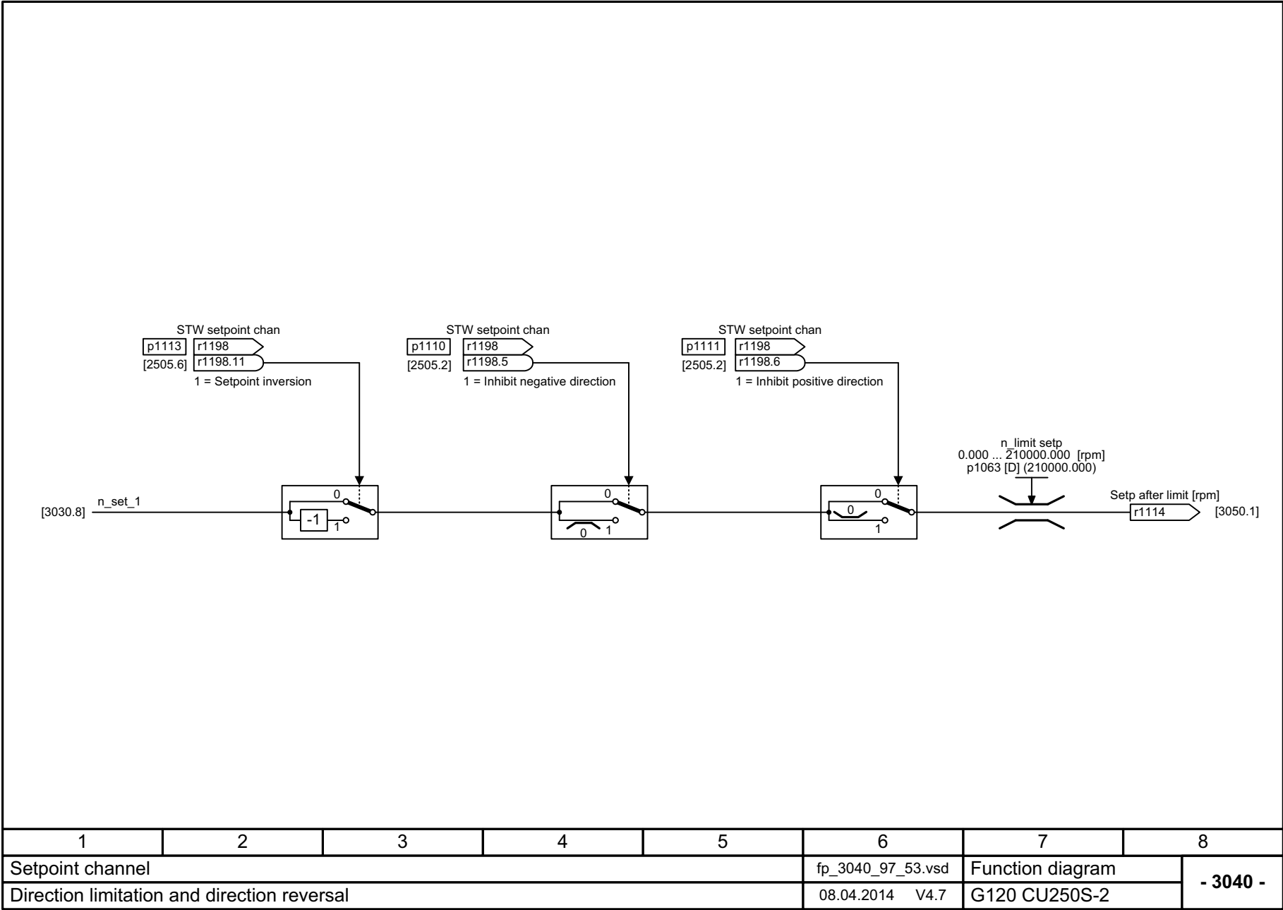
图 3-99 3040 - 方向限制和换向
