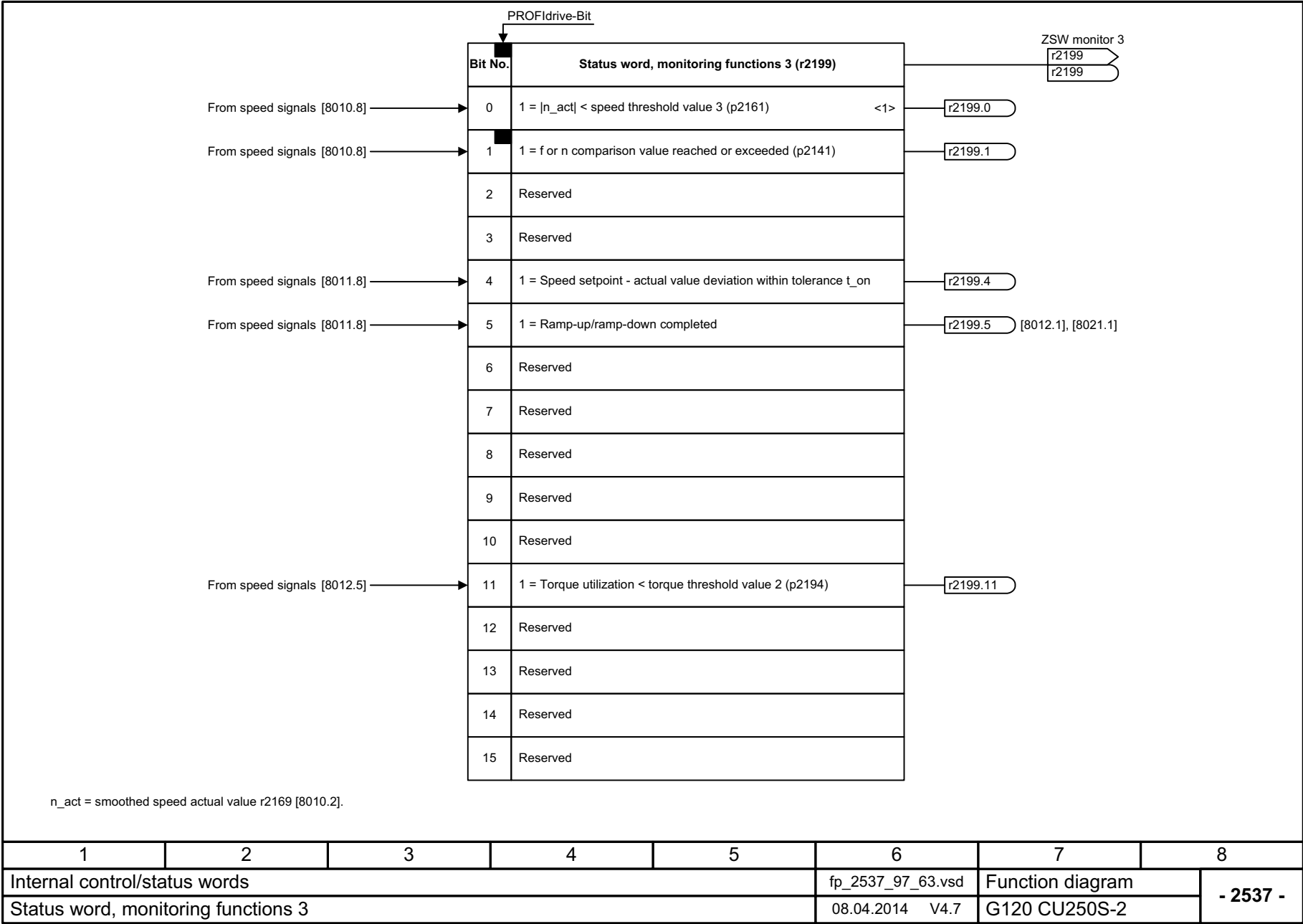
图 3-69 2537 - 监控 3 状态字
