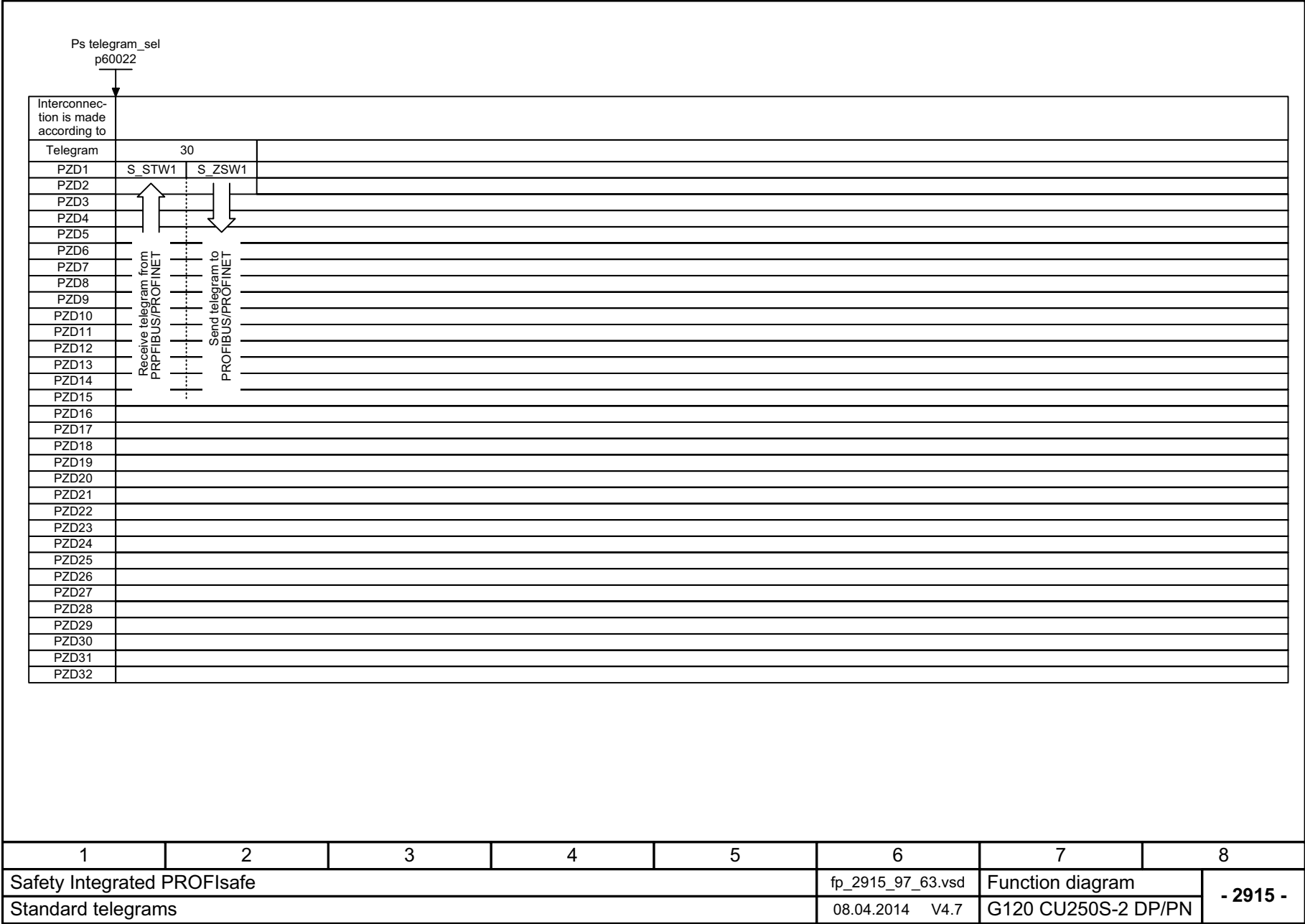
图 3-92 2915 - 标准报文
