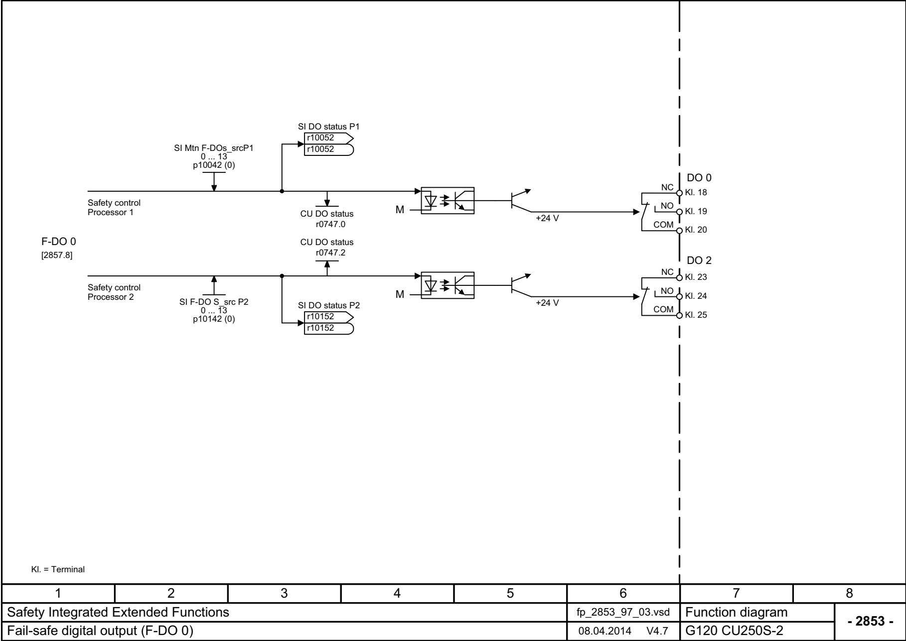
图 3-87 2853 - 故障安全数字输出端 (F-DO 0)
