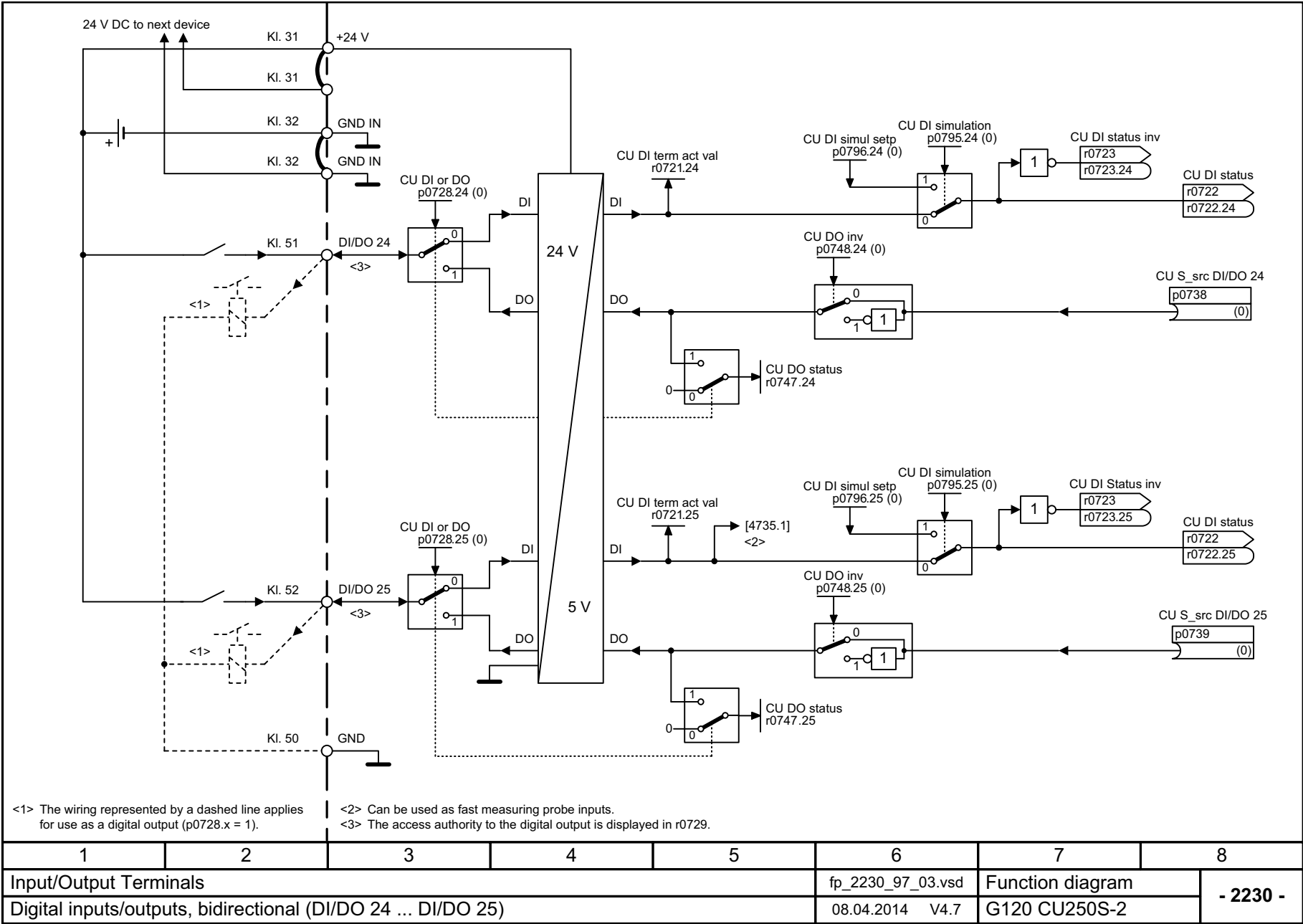
图 3-8 2230 - 双向数字输入端 / 输出端 (DI/DO 24 ... DI/DO 25)
