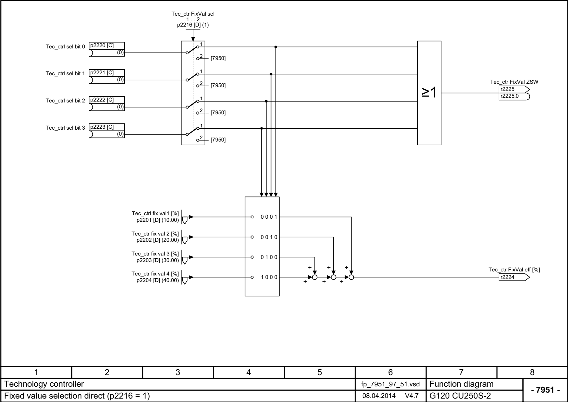
图 3-177 7951 - 固定值, 直接选择 (p2216 = 1)
