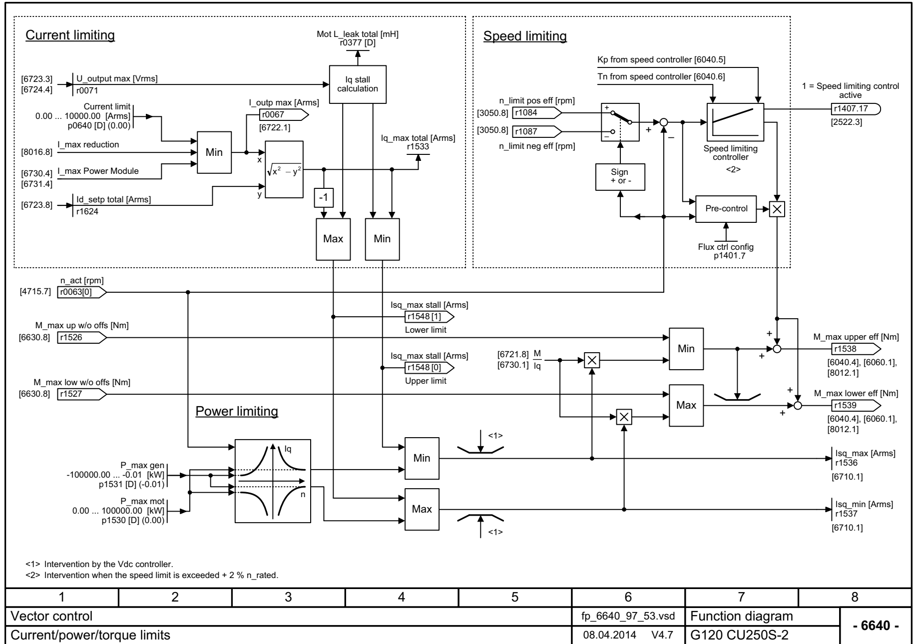
图 3-144 6640 - 电流极限 / 功率极限 / 转矩极限
