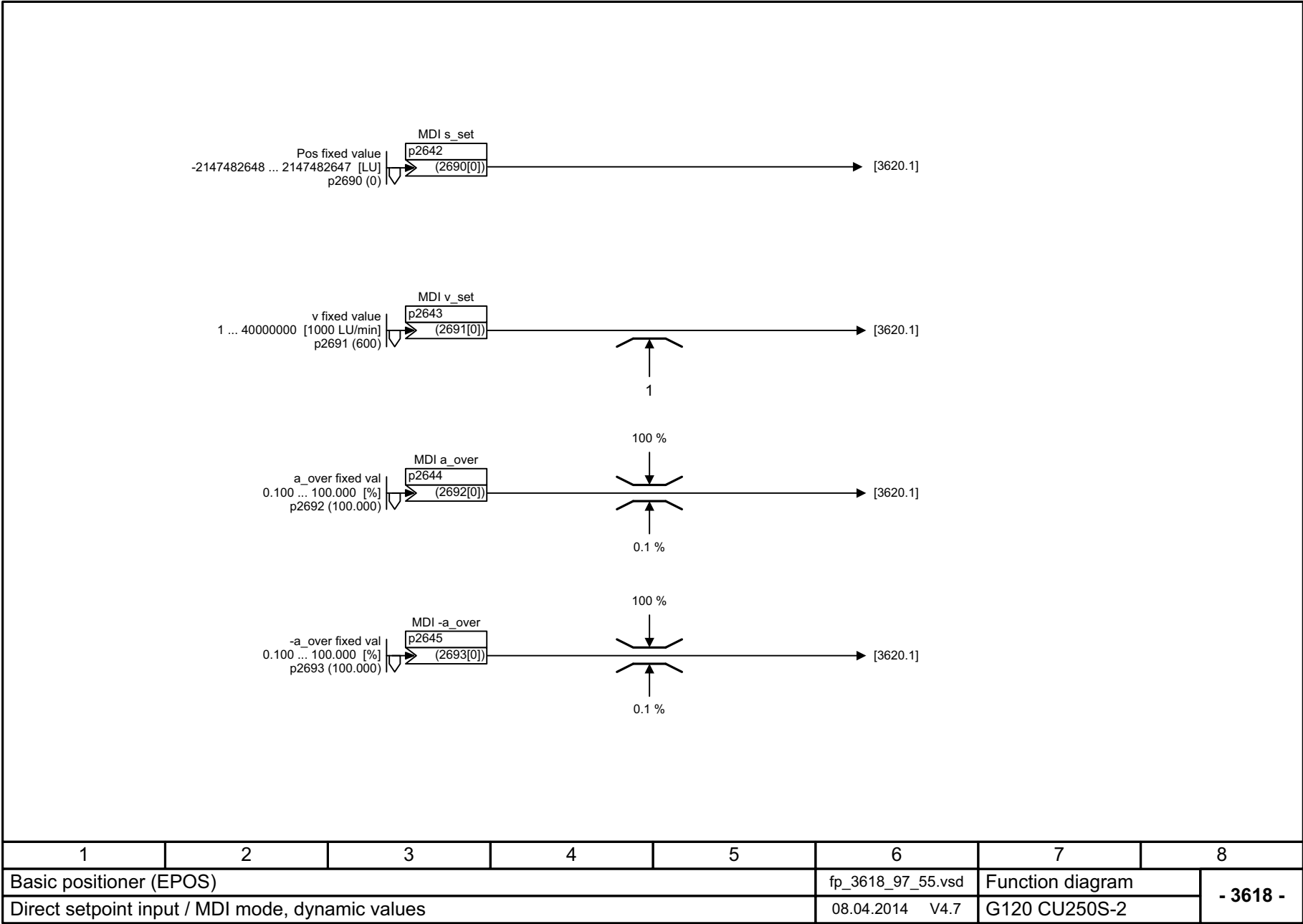
图 3-111 3618 - 设定值直接给定 / MDI, 动态值运行方式
