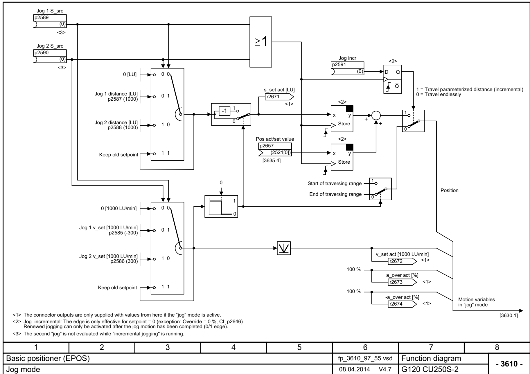
图 3-105 3610 - Jog 运行方式
