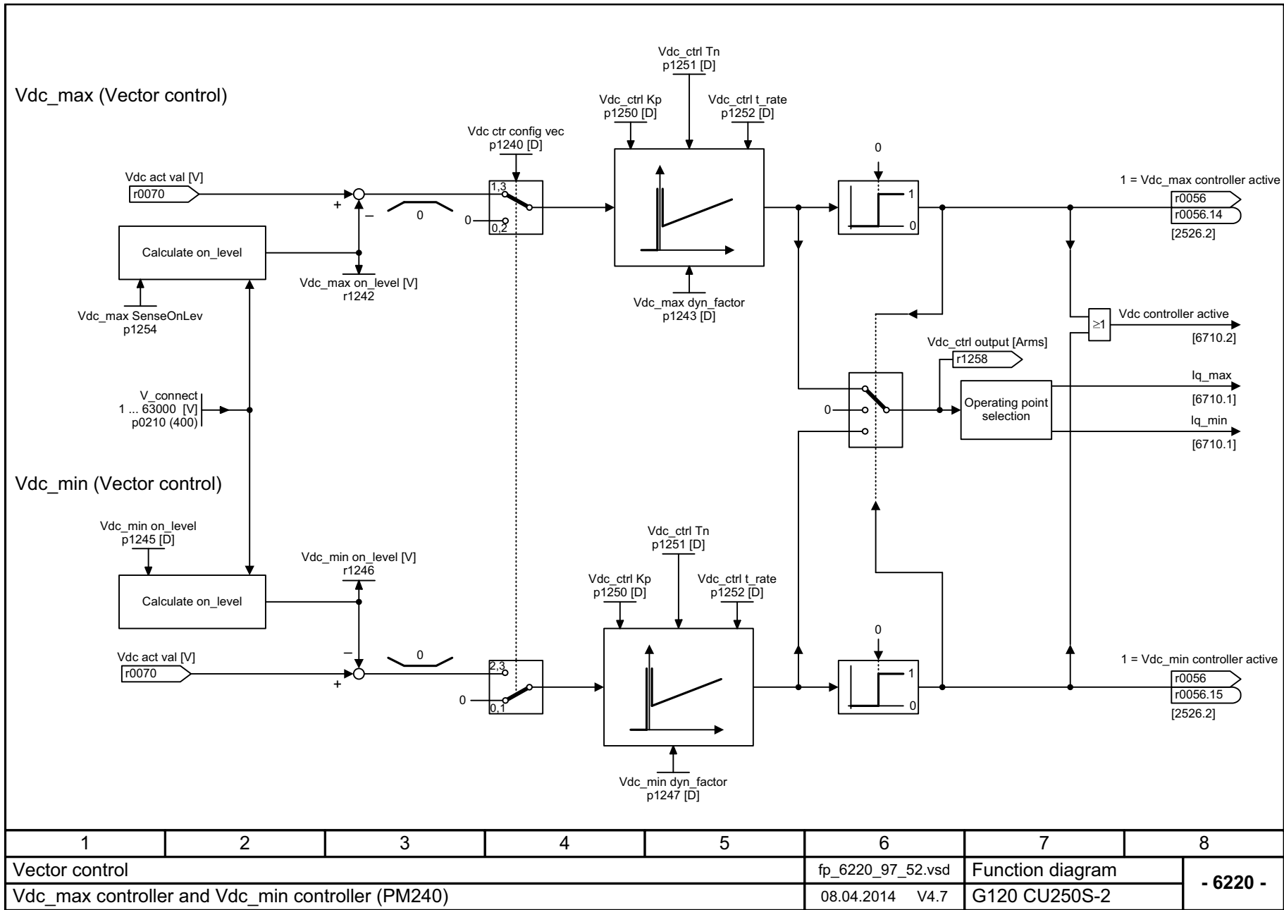
图 3-136 6220 - Vdc_max 控制器和 Vdc_min 控制器 (PM240)
