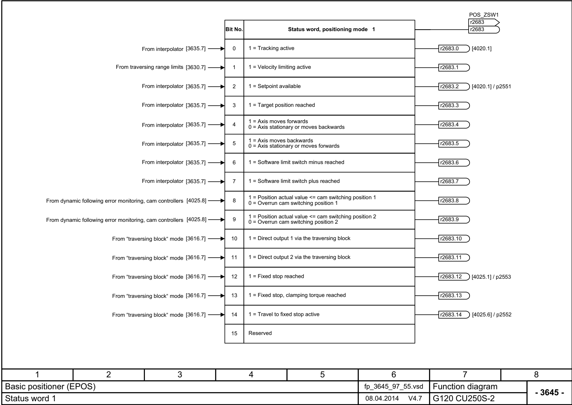
图 3-117 3645 - 状态字 1
