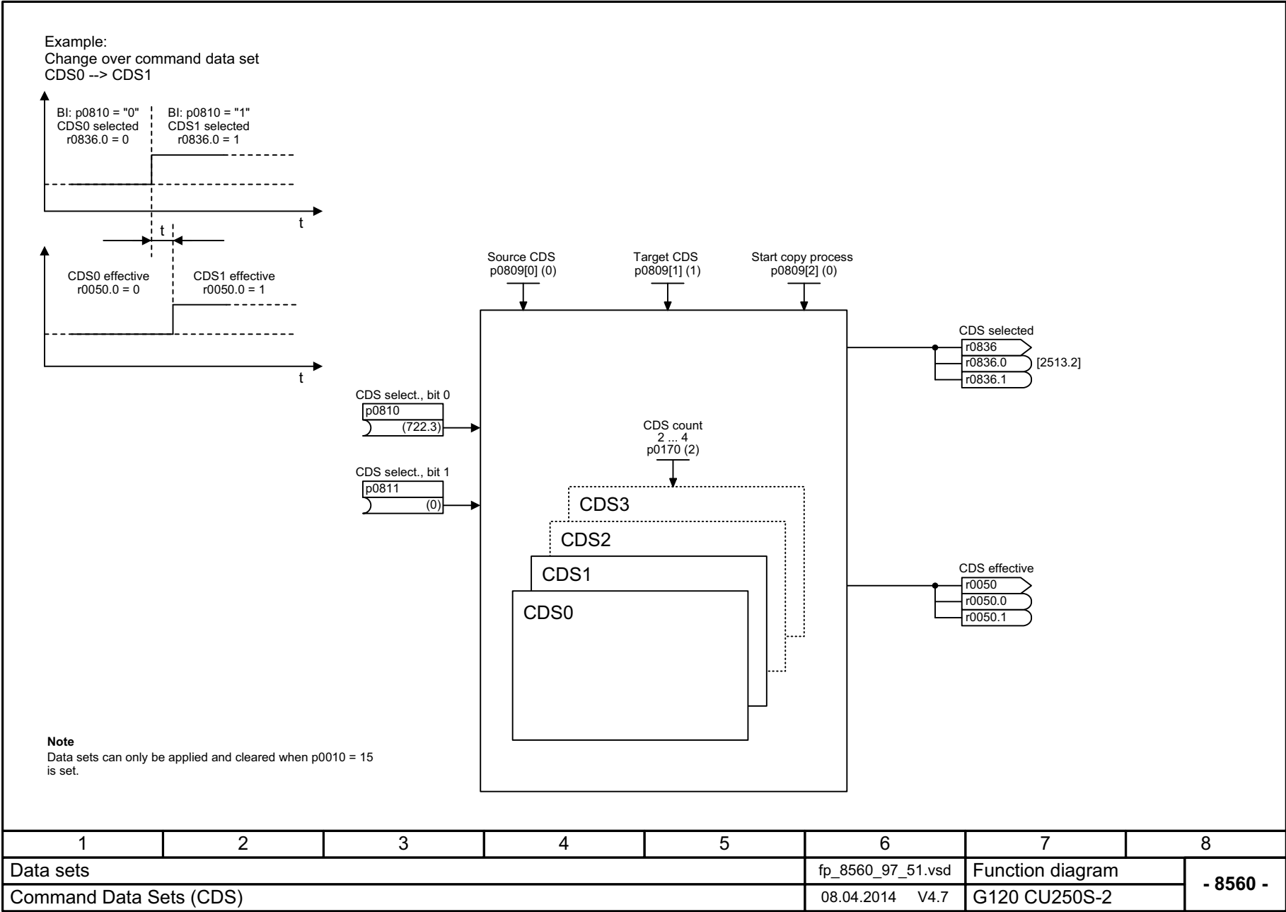
图 3-195 8560 - 指令数据组 (Command Data Set, CDS)
