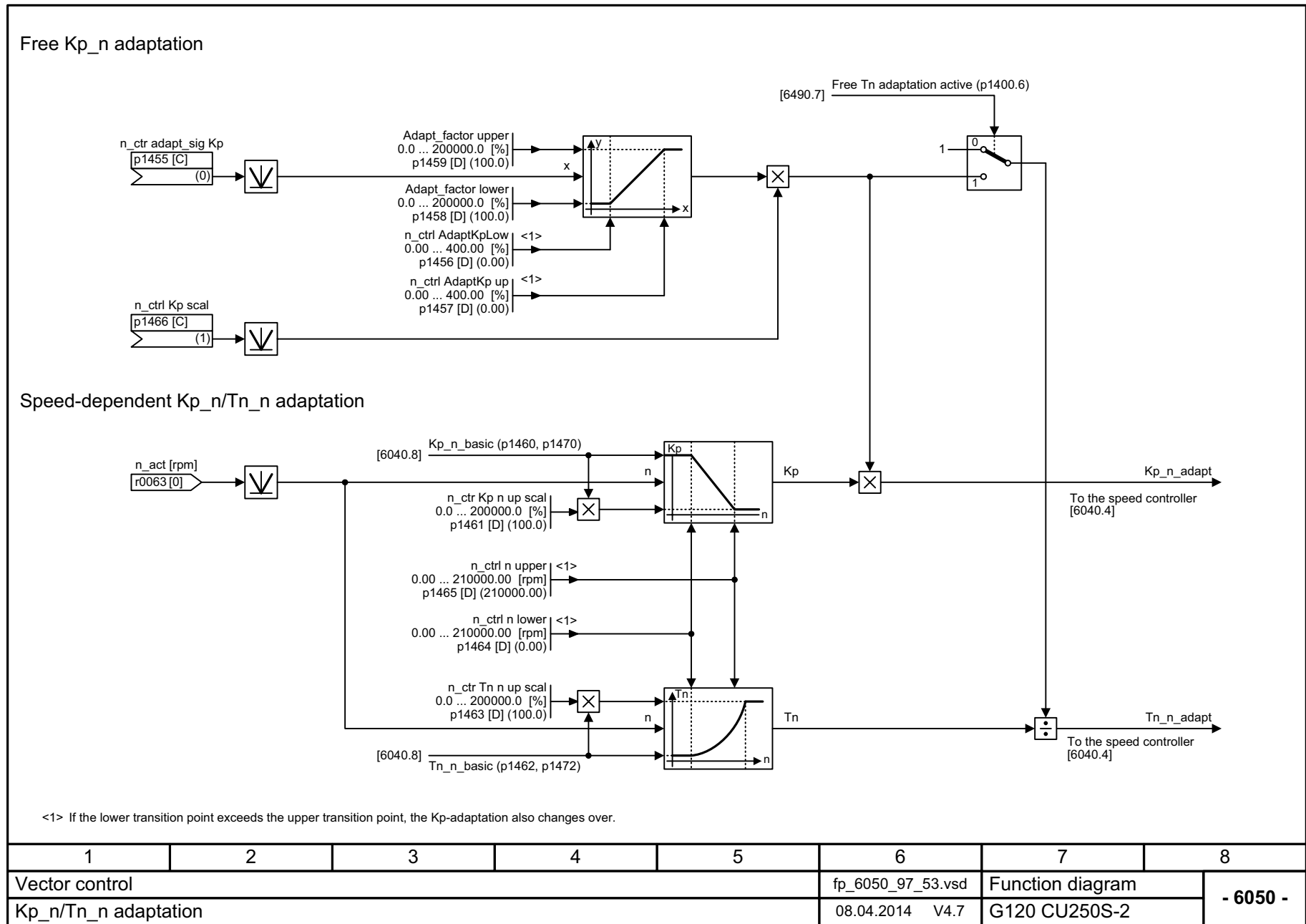
图 3-134 6050 - Kp_n-/Tn_n 适配
