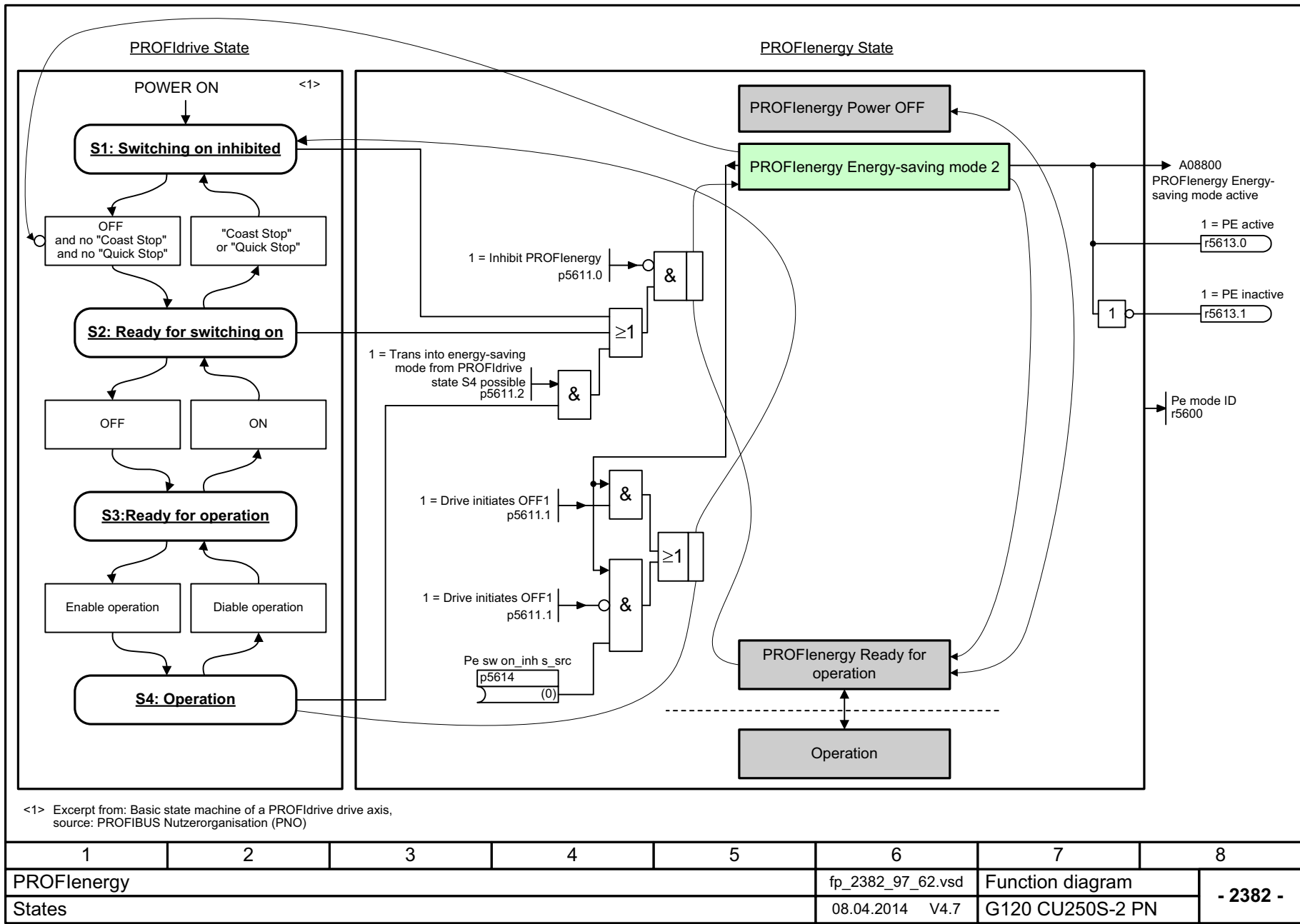
图 3-16 2382 - 状态
