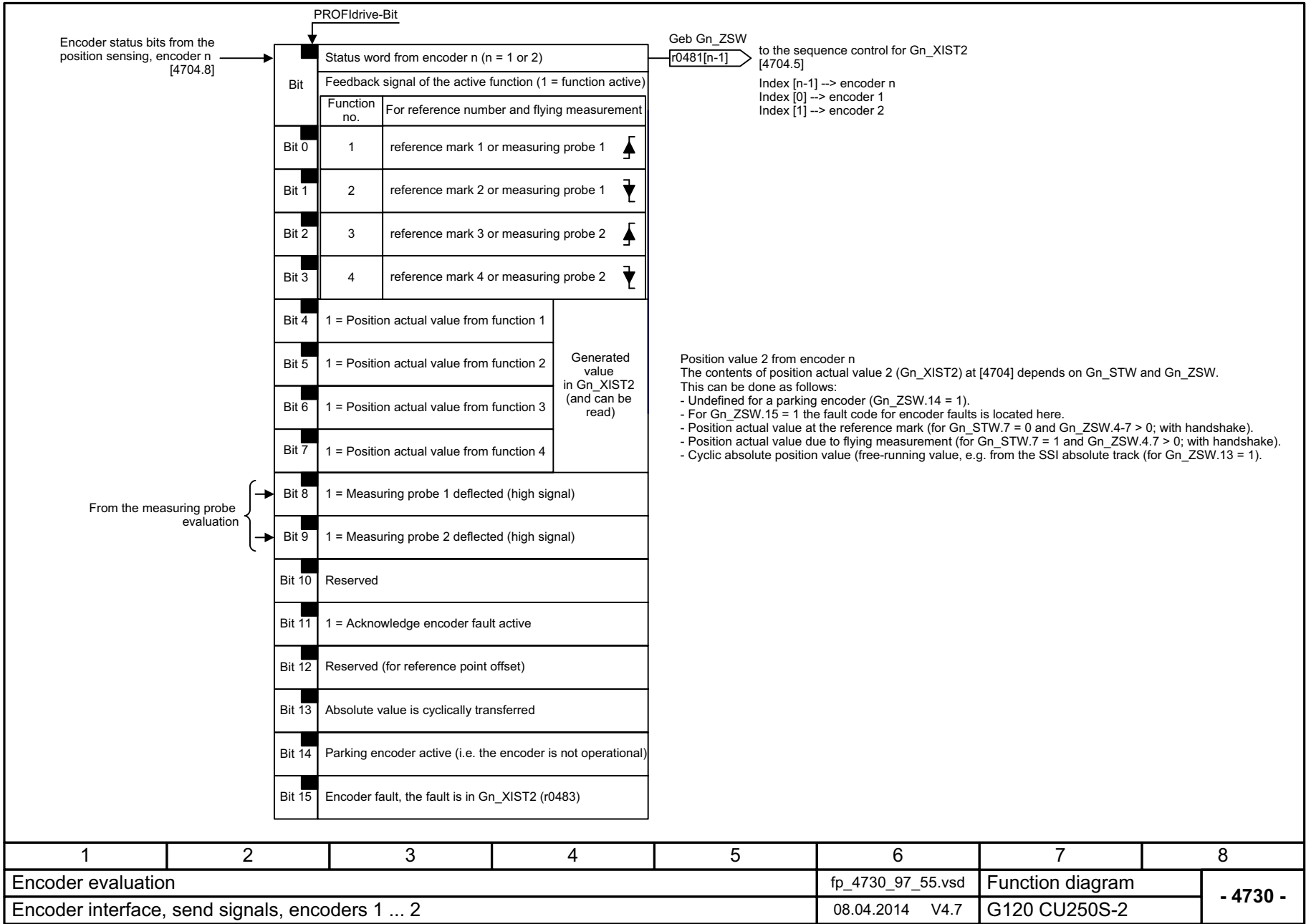
图 3-127 4730 - 编码器接口, 发送信号编码器 1 ... 2
