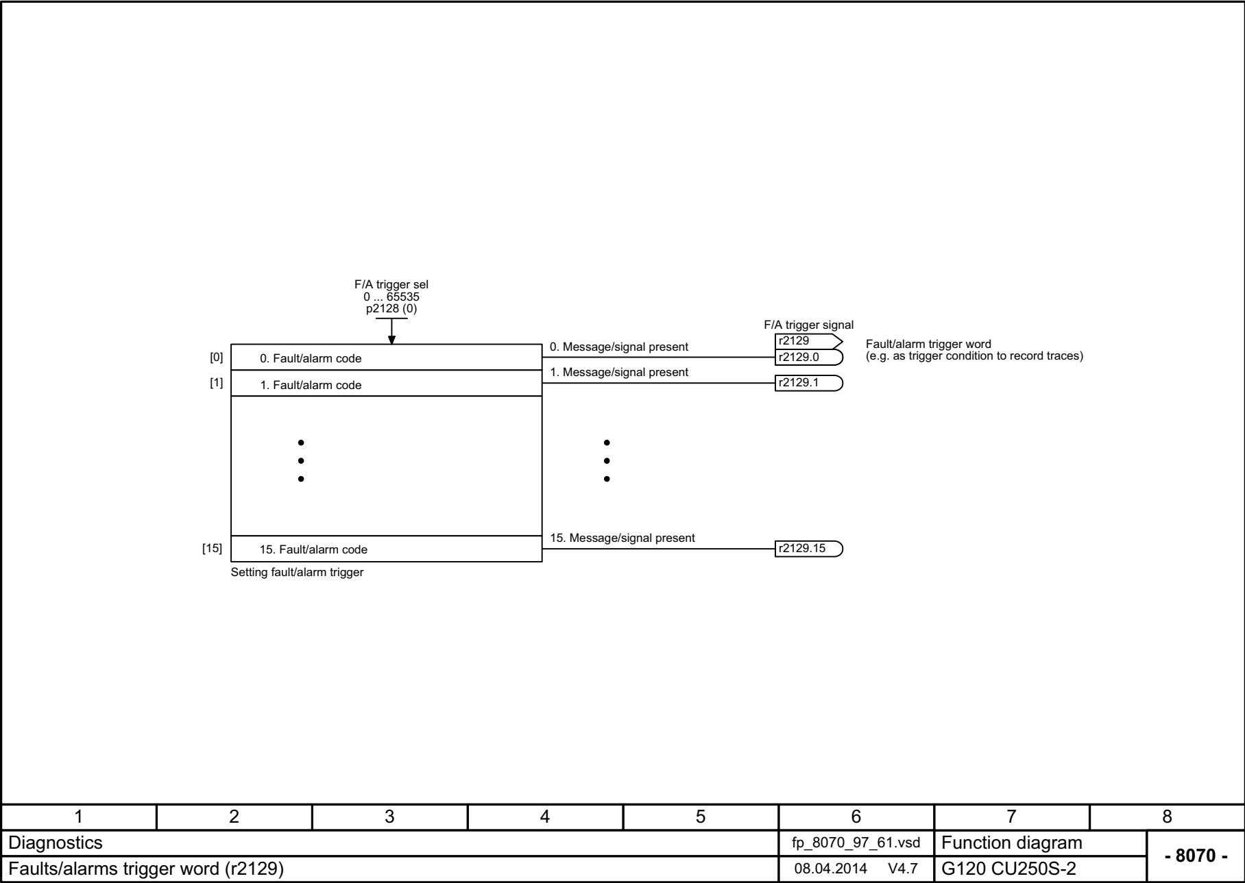
图 3-193 8070 - 故障 / 报警触发字 (r2129)
