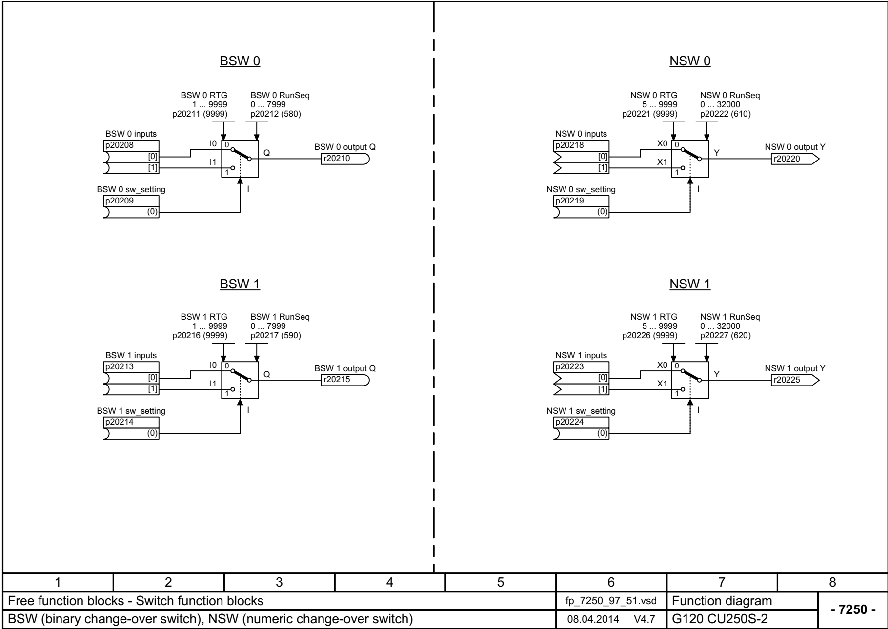
图 3-171 7250 - BSW (二进制转换器), NSW (数字转换器)
