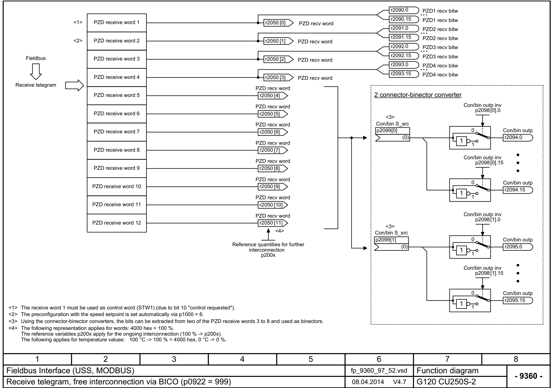
图 3-53 9360 - 通过 BICO 自由互连接收报文 (p0922 = 999)
