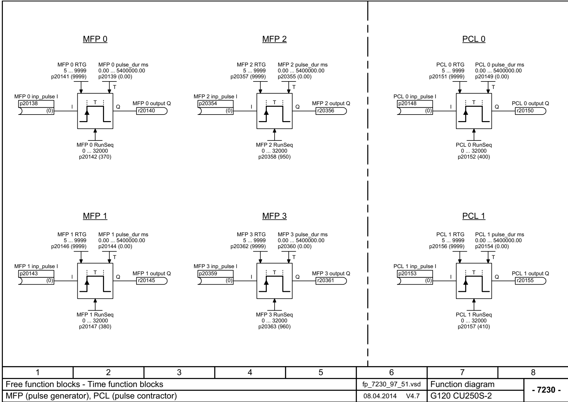
图 3-166 7230 - MFP (脉冲发生器), PCL (脉冲缩短器)
