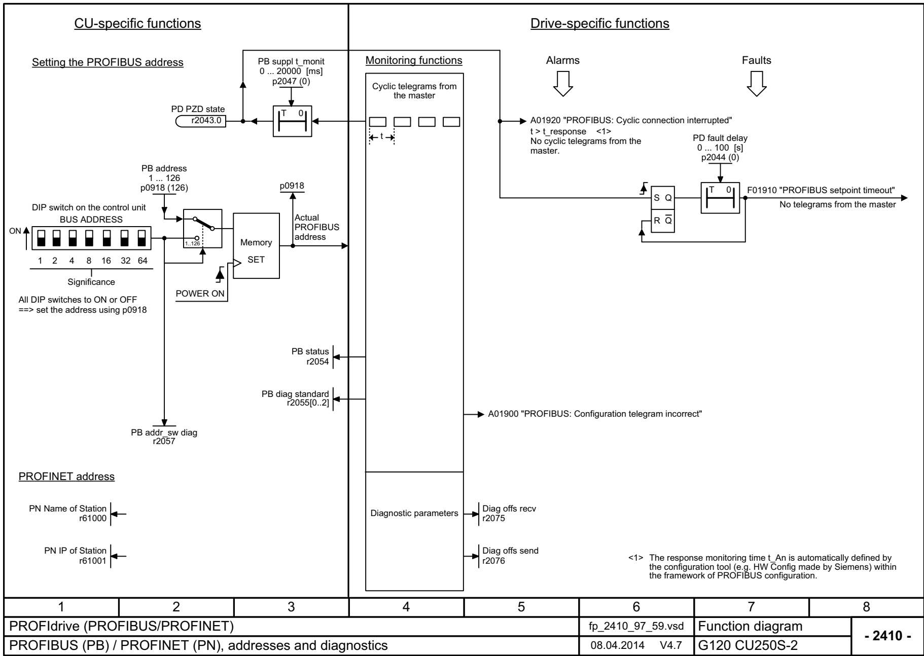
图 3-18 2410 - PROFIBUS (PB) / PROFINET (PN), 地址和诊断
