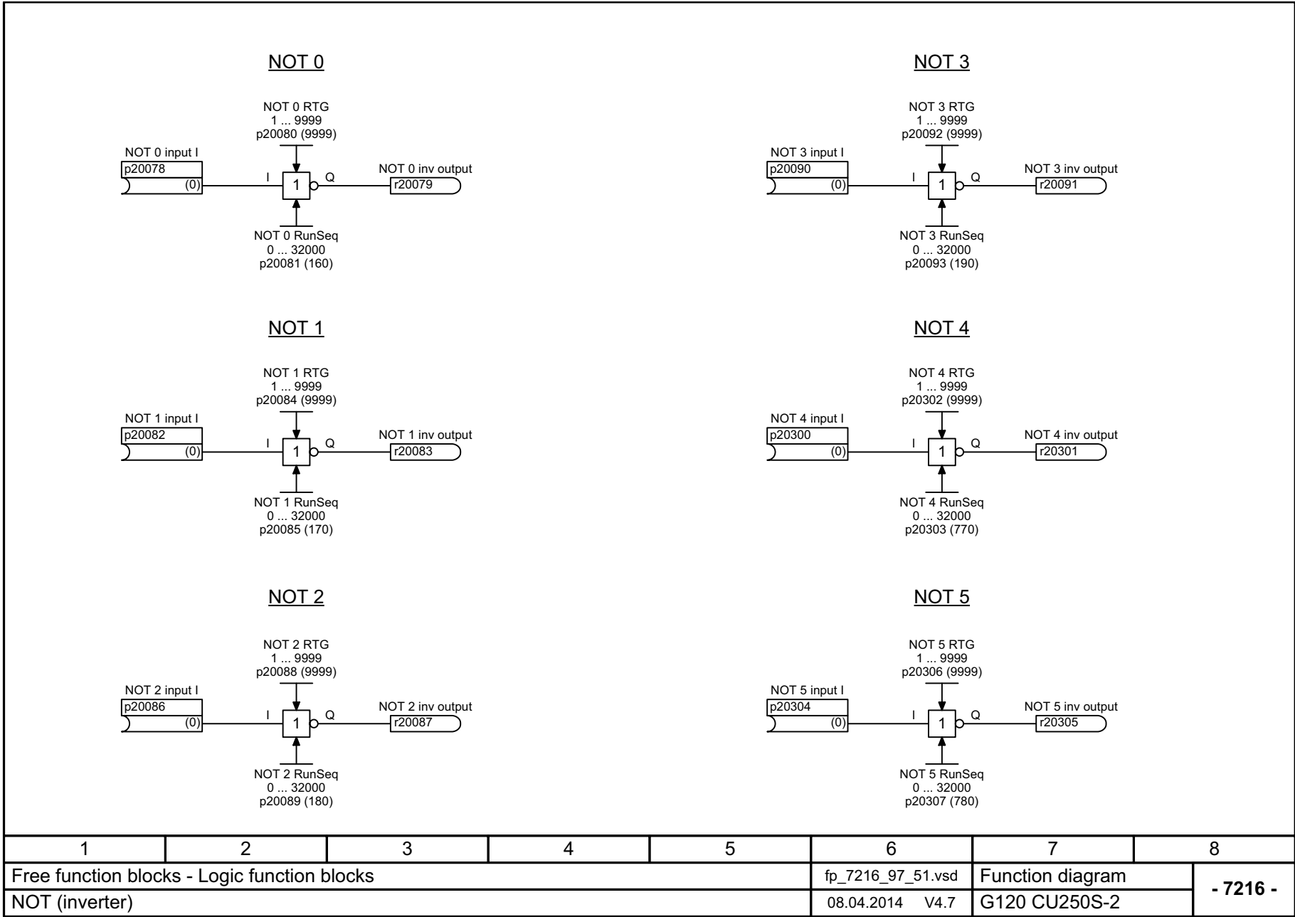
图 3-160 7216 - NOT (非)
