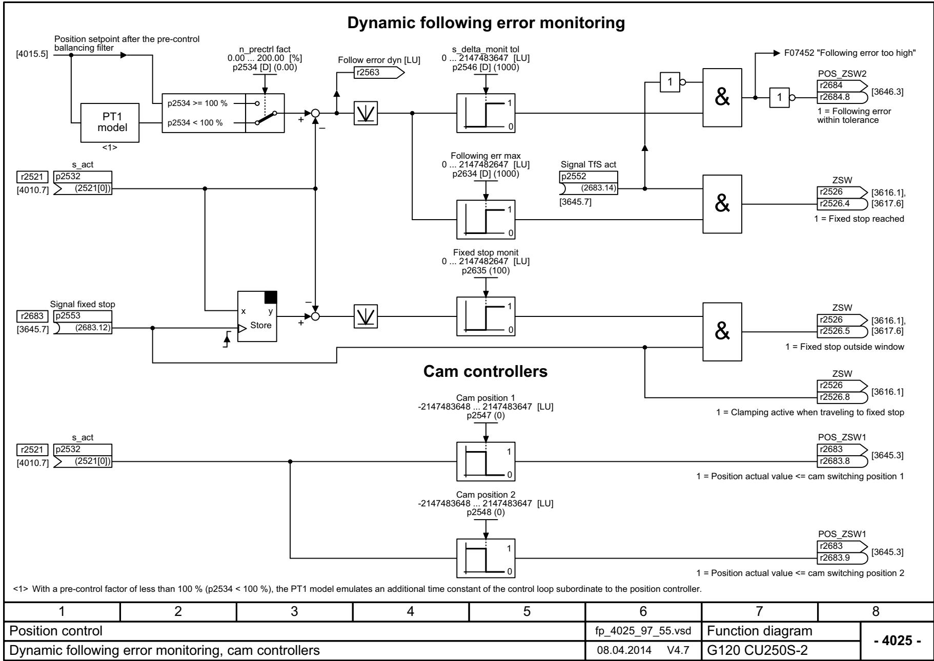
图 3-123 4025 - 动态滞后量监控, 凸轮开关
