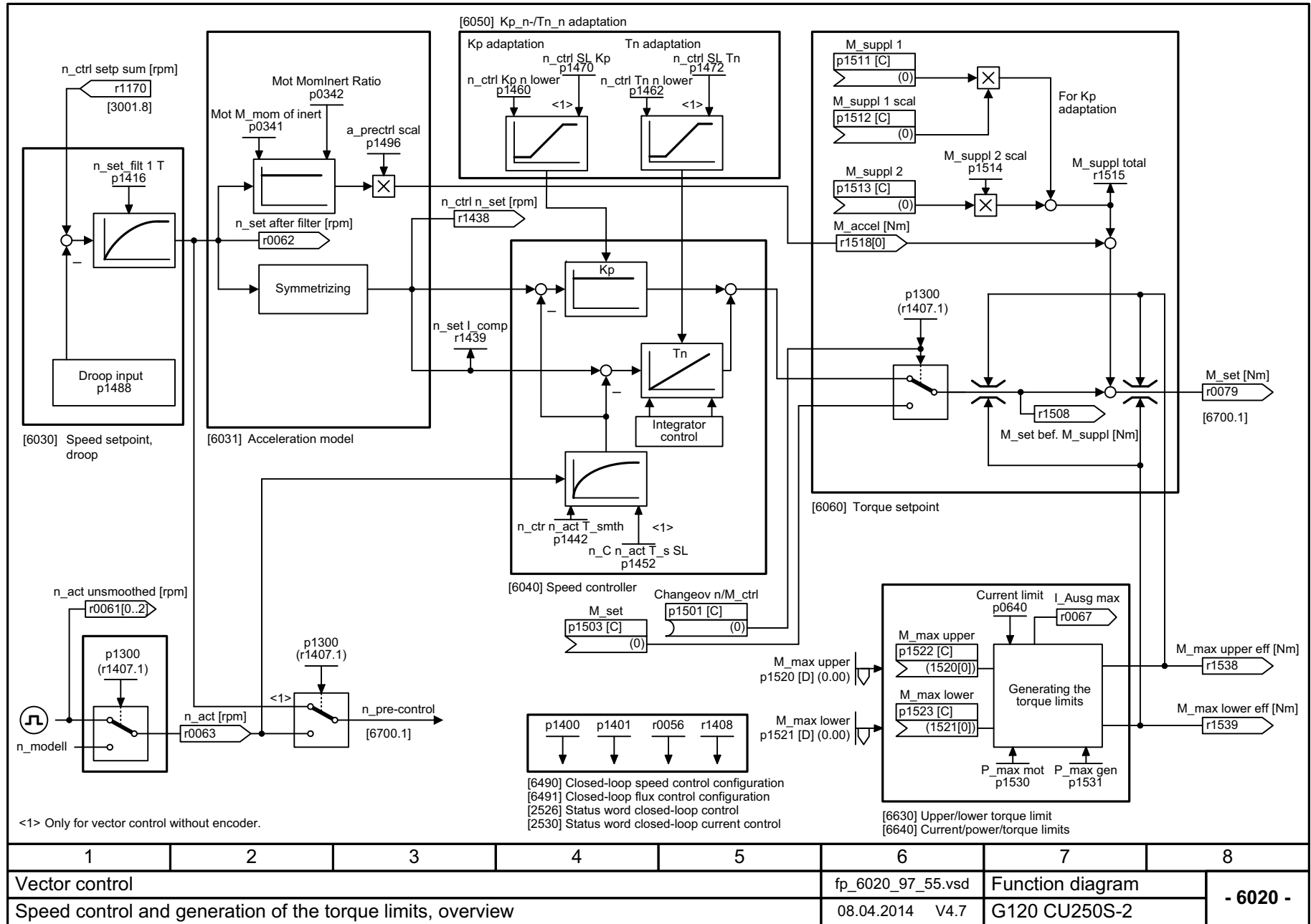
图 3-130 6020 - 转速控制和转矩限值形成, 一览
