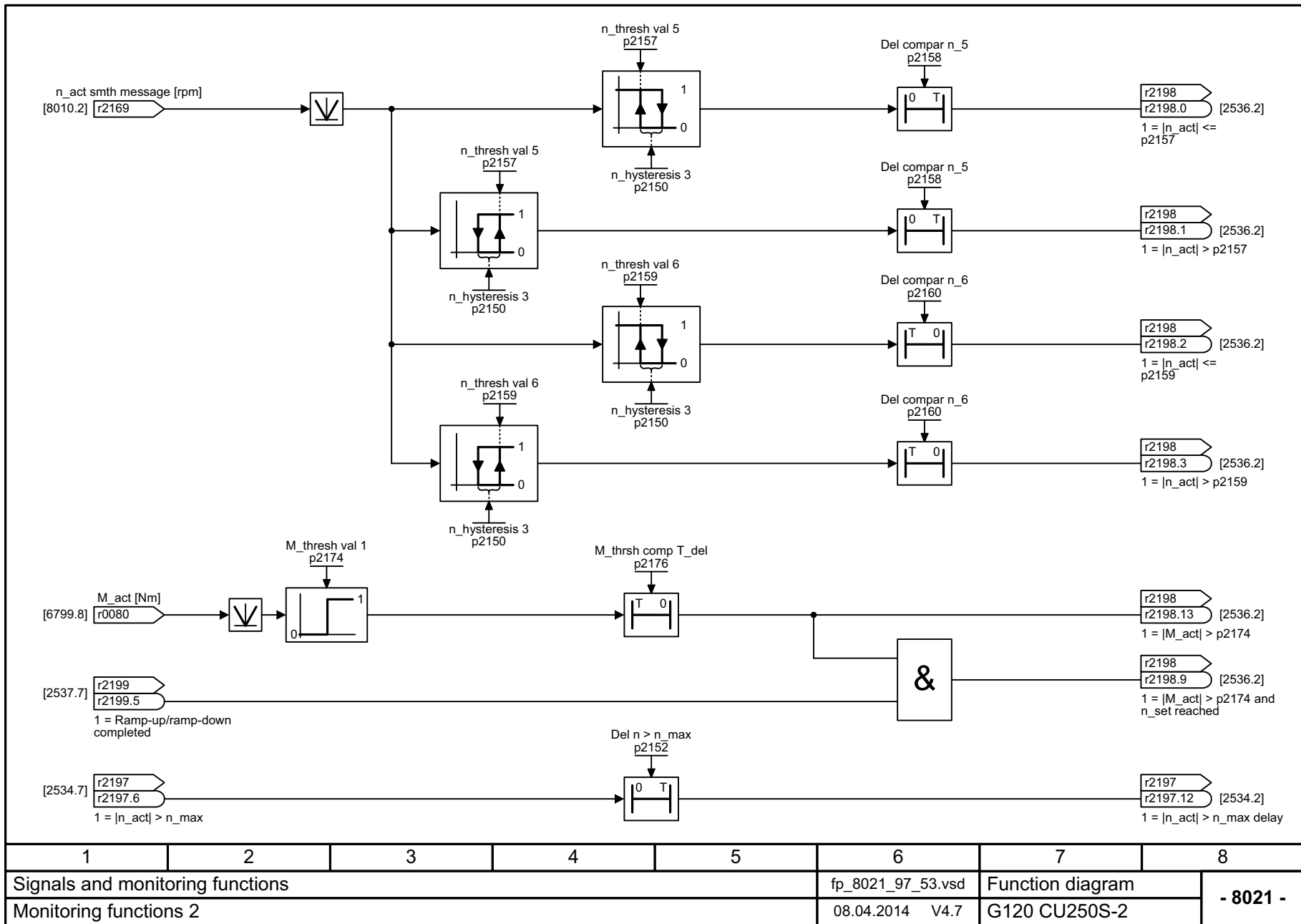
图 3-189 8021 - 监控功能 2
