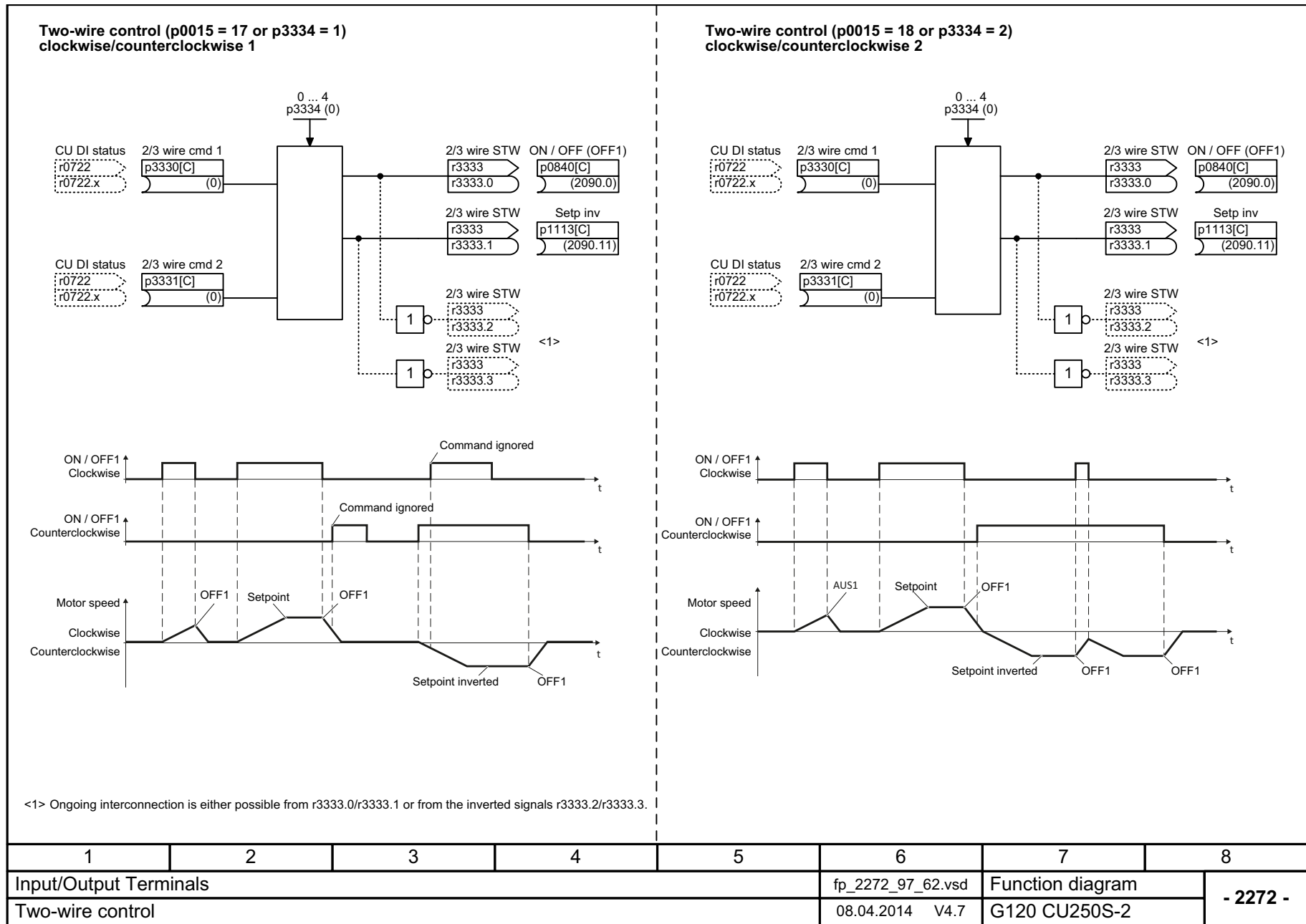
图 3-13 2272 - 双线制控制
