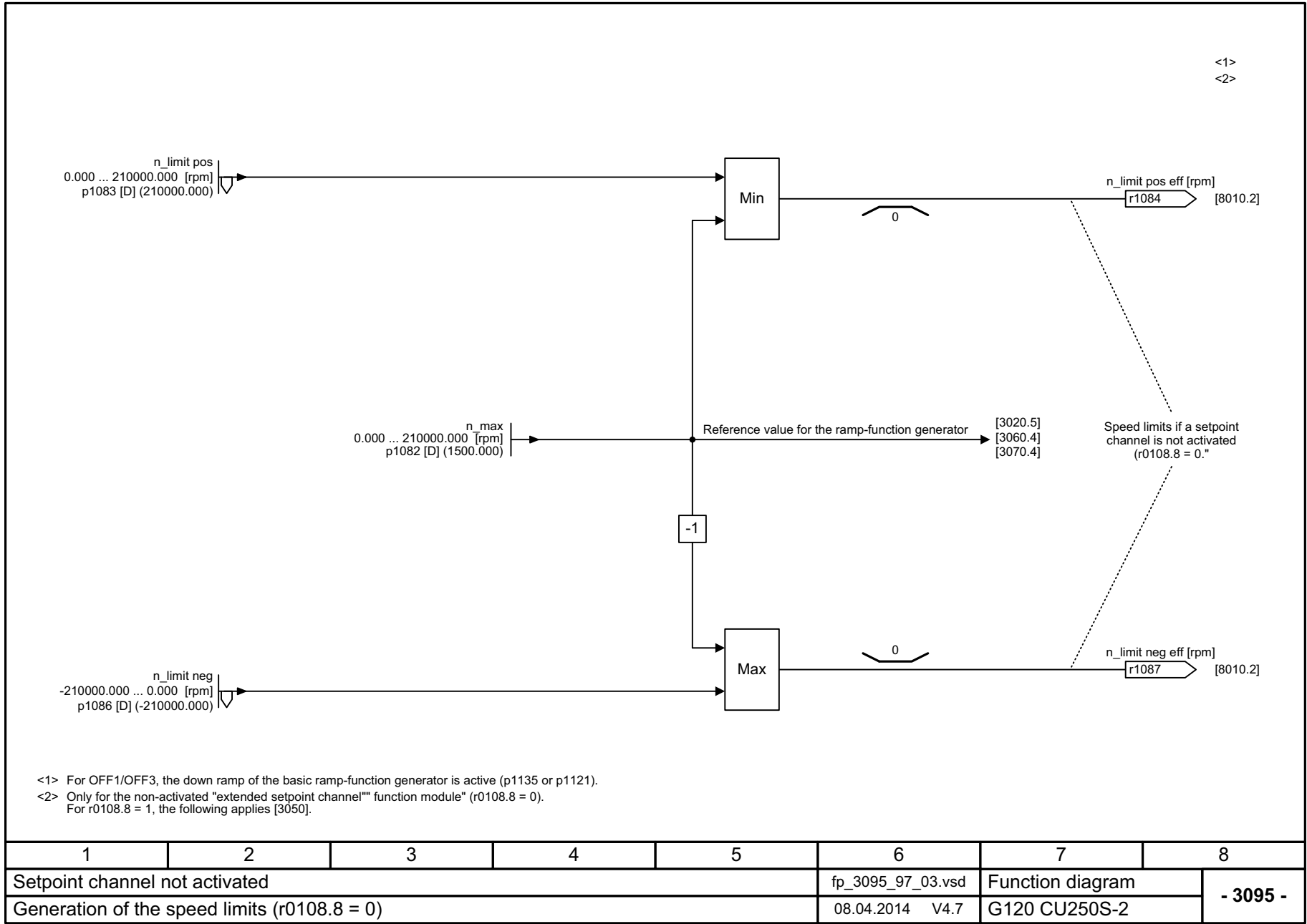
图 3-104 3095 - 转速极限值形成 (r0108.8 = 0)
