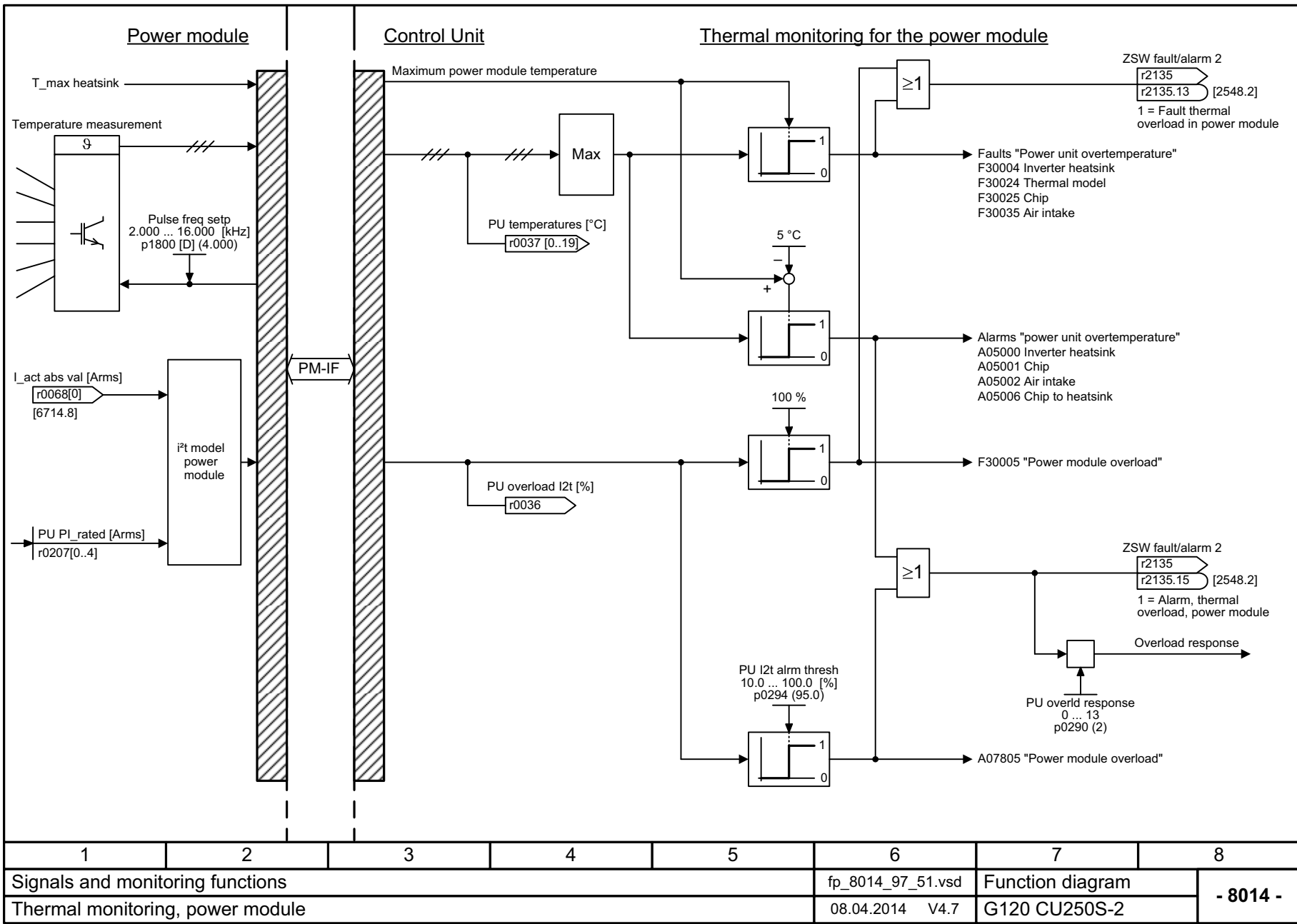
图 3-185 8014 - 功率单元热负荷监控
