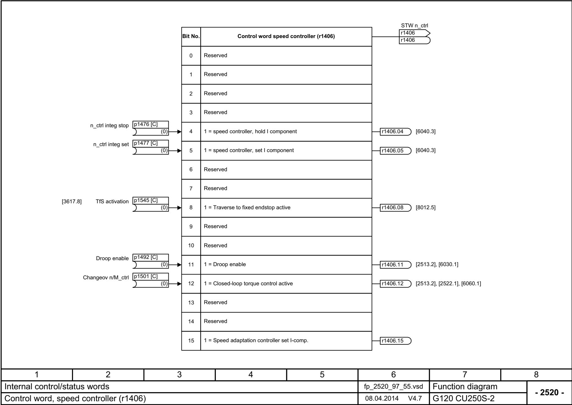
图 3-63 2520 - 转速控制器控制字 (r1406)
