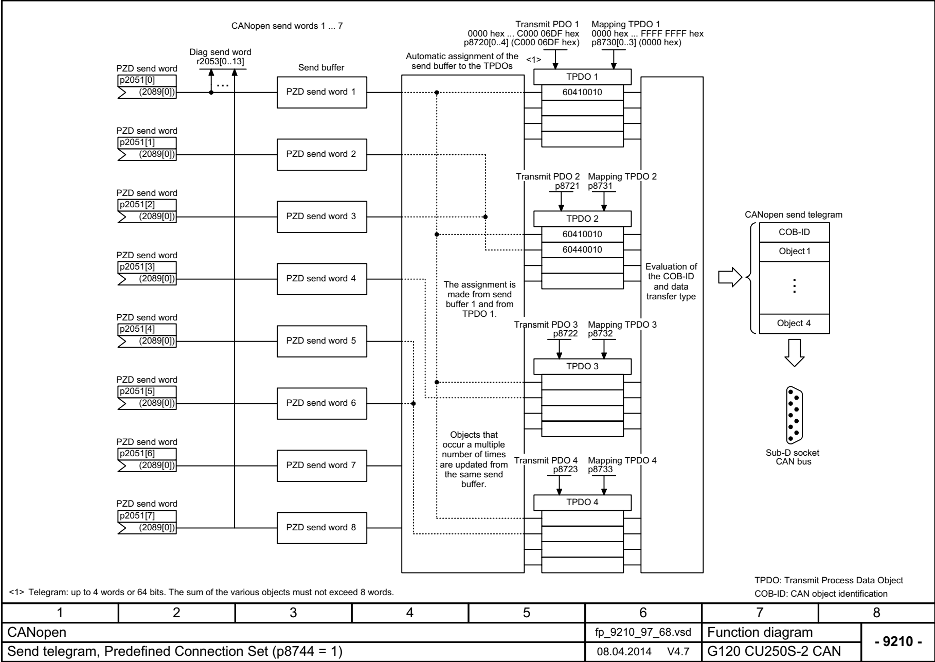
图 3-47 9210 - 预定义连接组发送报文 (p8744 = 1)
