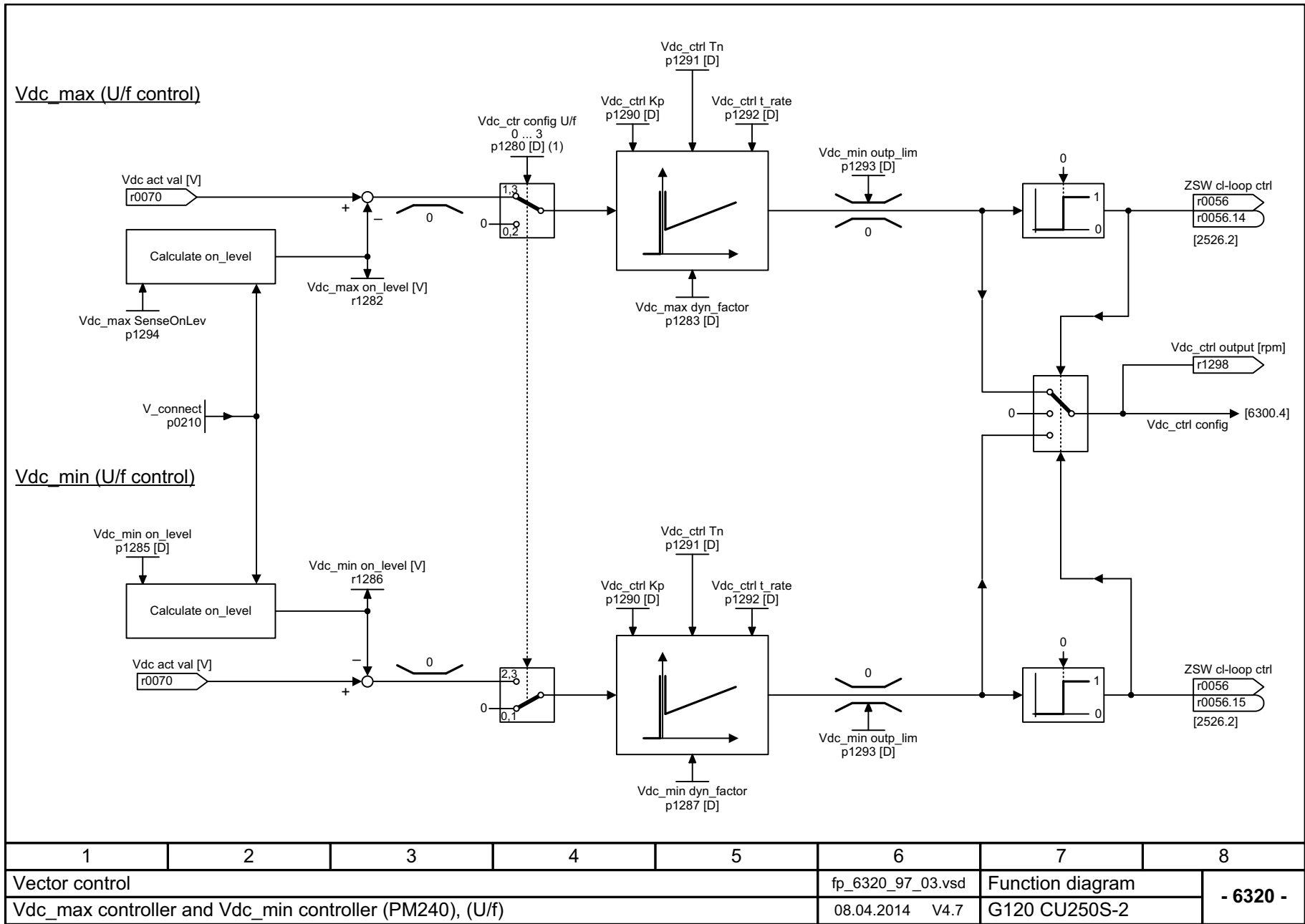
图 3-140 6320 - Vdc_max 控制器和 Vdc_min 控制器 (PM240), (V/f)
