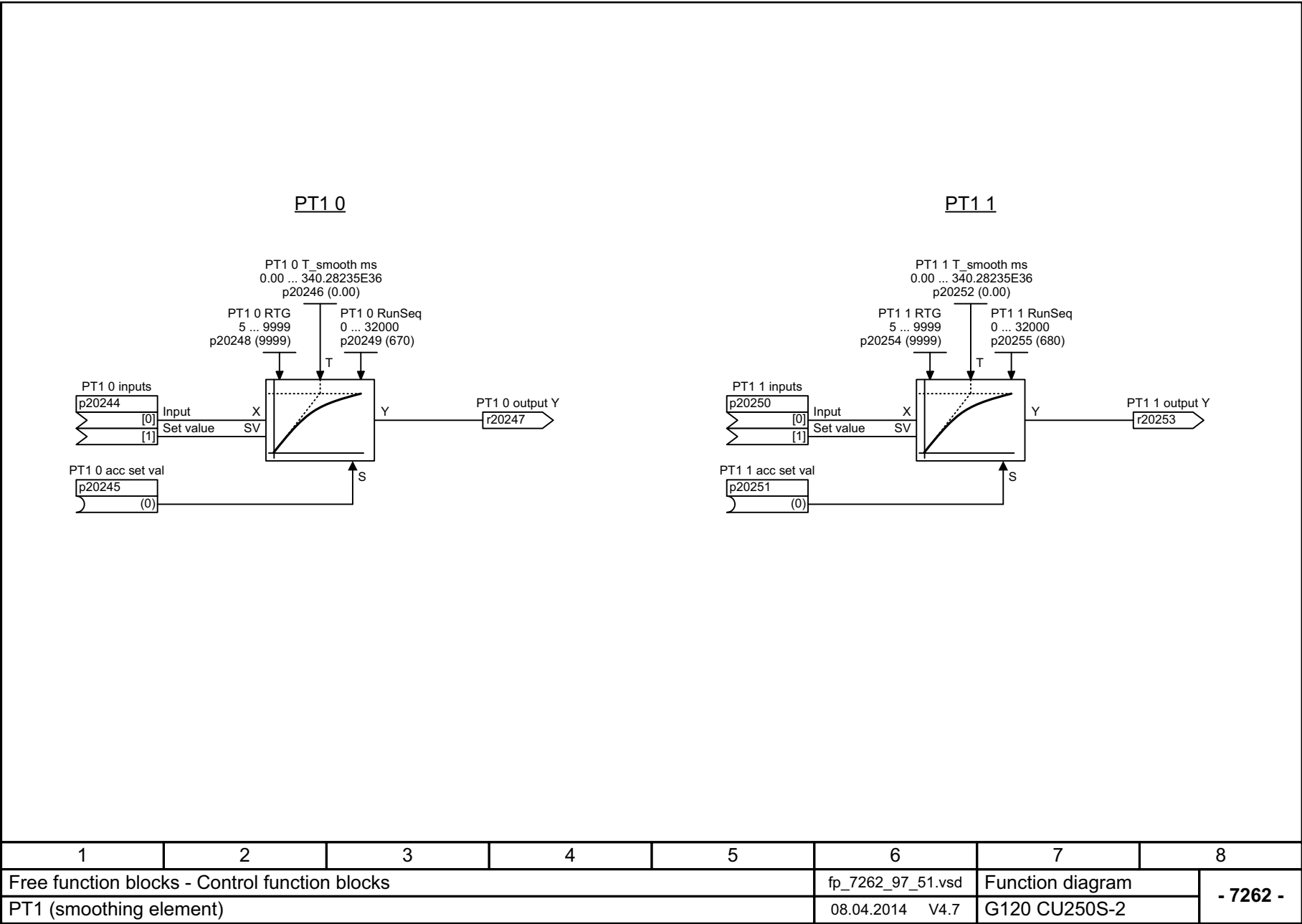
图 3-173 7262 - PT1 (平滑元件)
