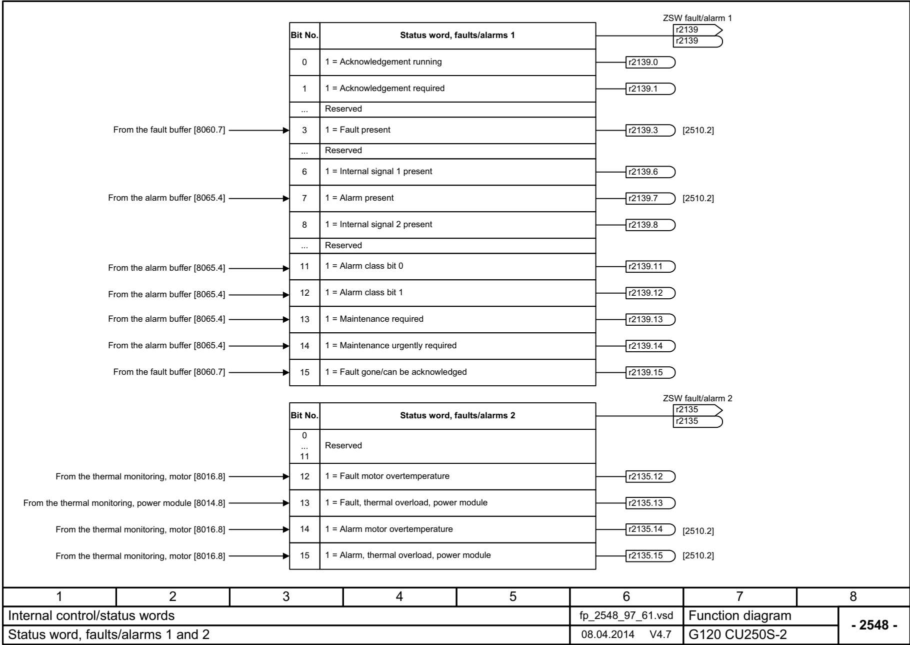
图 3-71 2548 - 故障 / 报警 1 和 2 状态字
