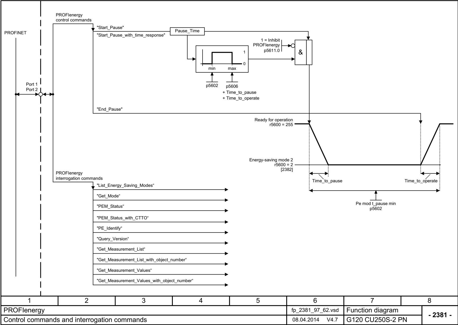
图 3-15 2381 - 控制指令和查询指令
