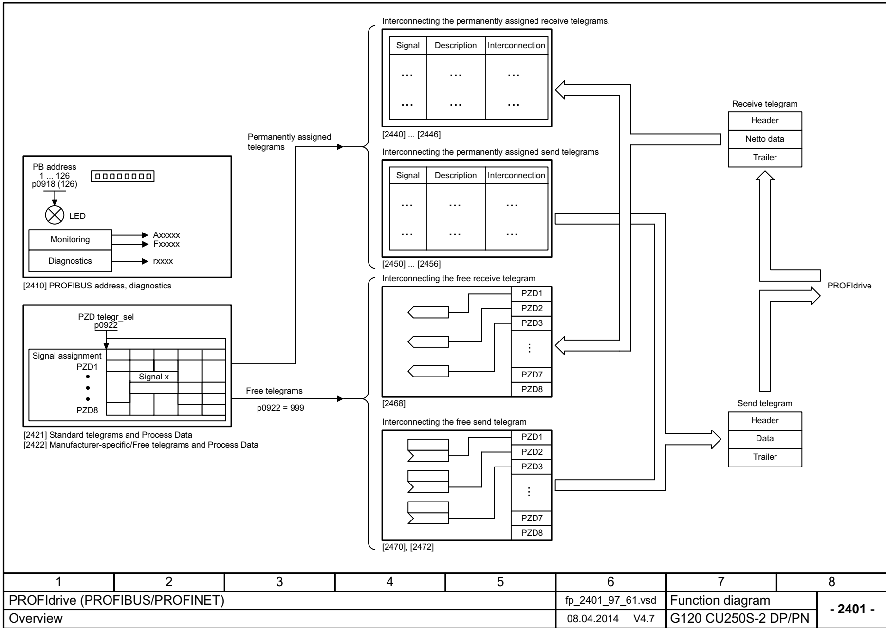
图 3-17 2401 - 一览
