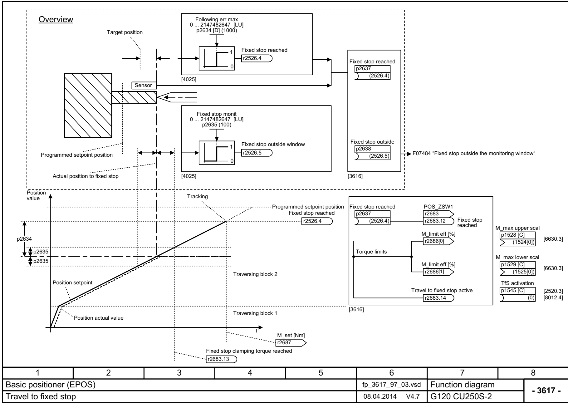
图 3-110 3617 - 运行到固定挡块
