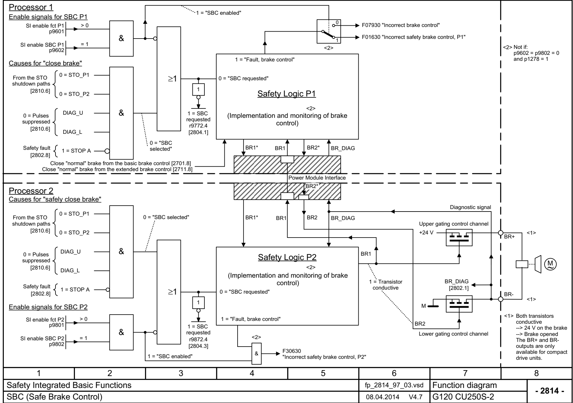
图 3-80 2814 - SBC (Safe Brake Control)
