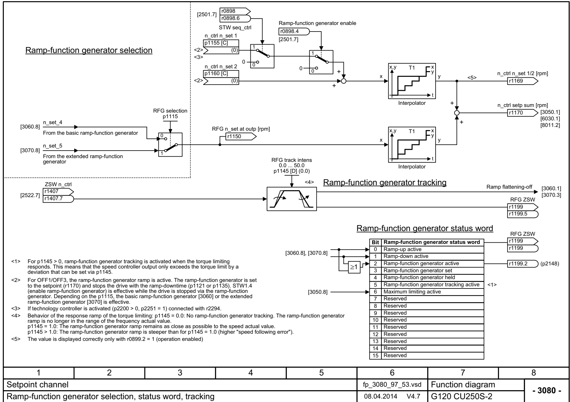
图 3-103 3080 - 斜坡函数发生器选择, 斜坡函数发生器状态字, 斜坡函数发生器跟踪
