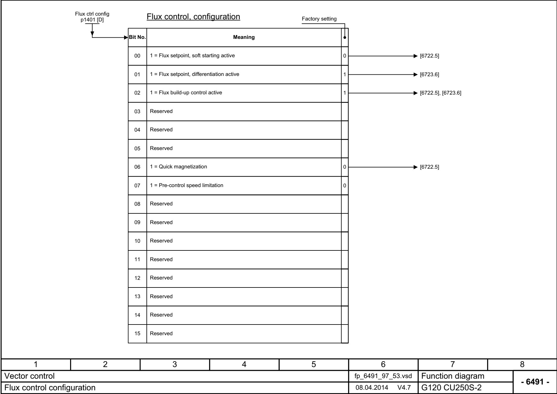
图 3-142 6491 - 磁通控制配置
