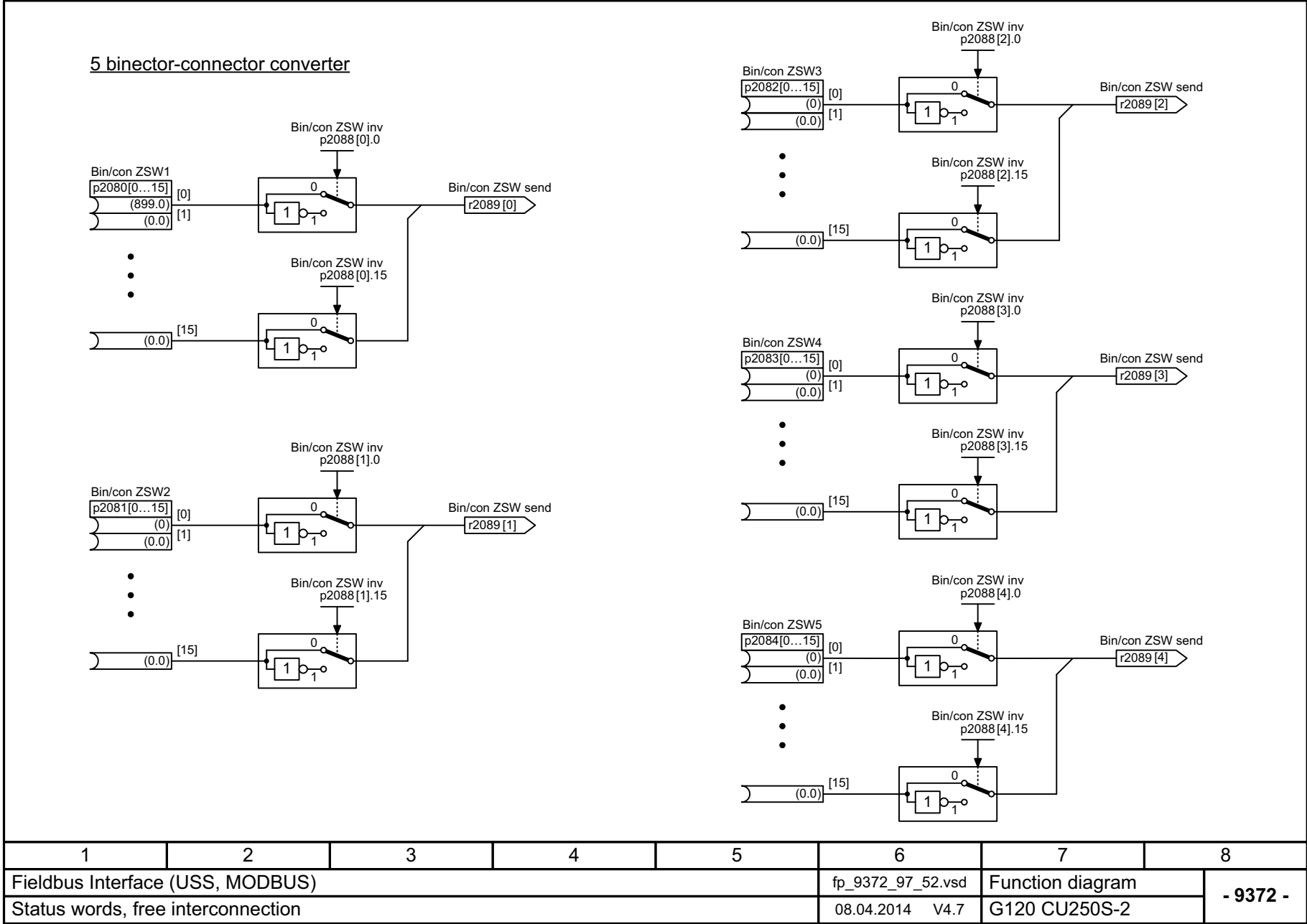
图 3-55 9372 - 自由互联状态字
