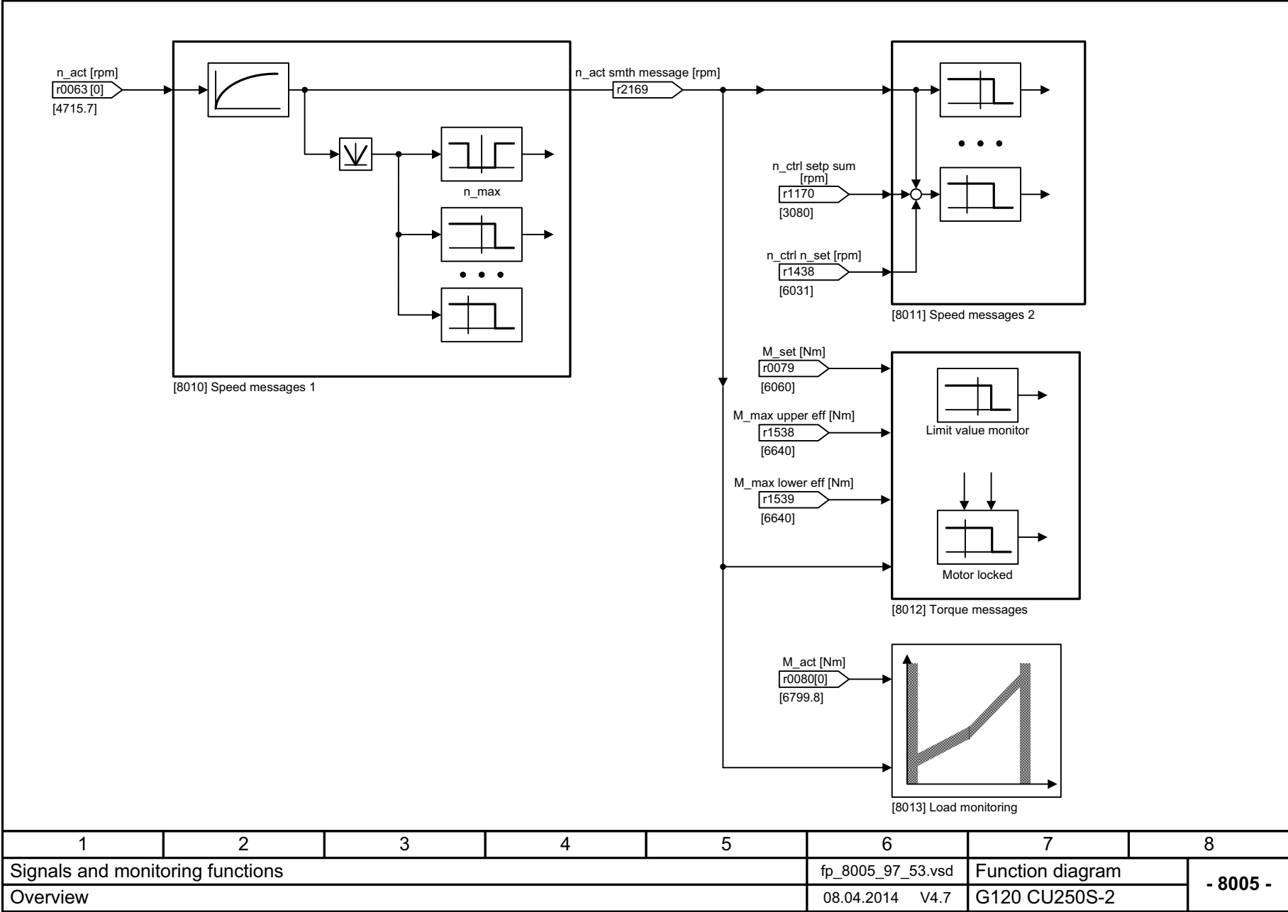
图 3-180 8005 - 一览
