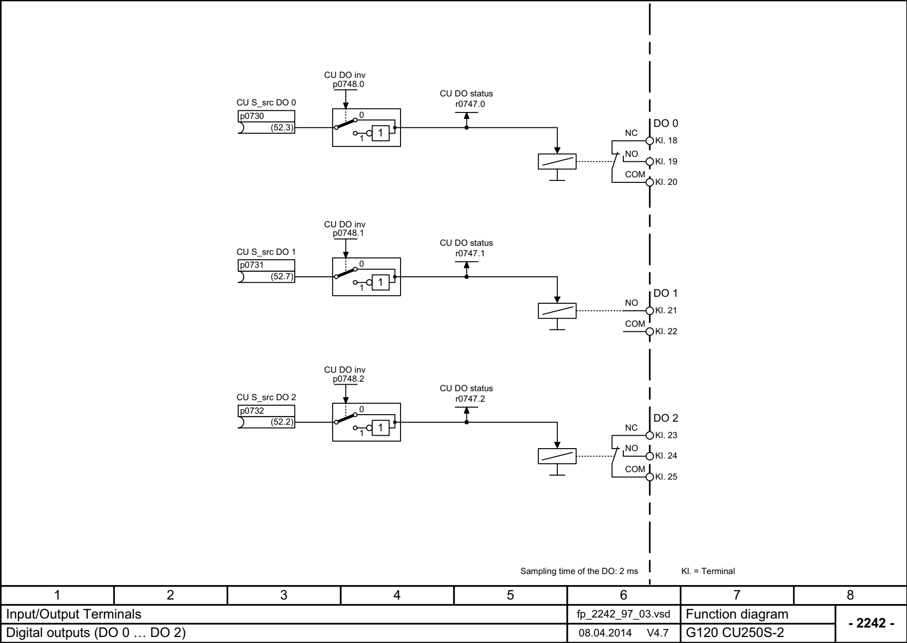
图 3-10 2242 - 数字输出端 (DO 0 ... DO 2)
