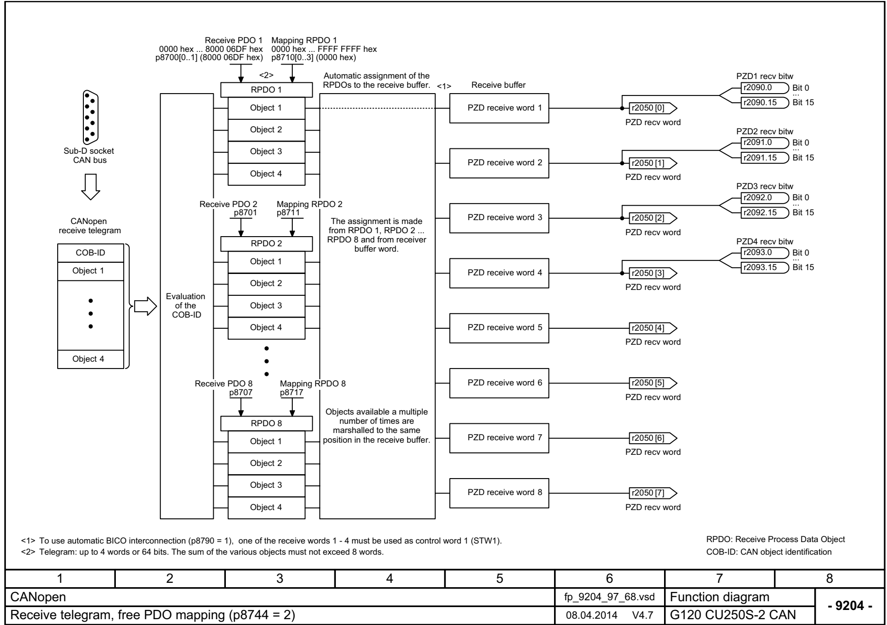
图 3-44 9204 - 自由 PDO 映射接收报文 (p8744 = 2)
