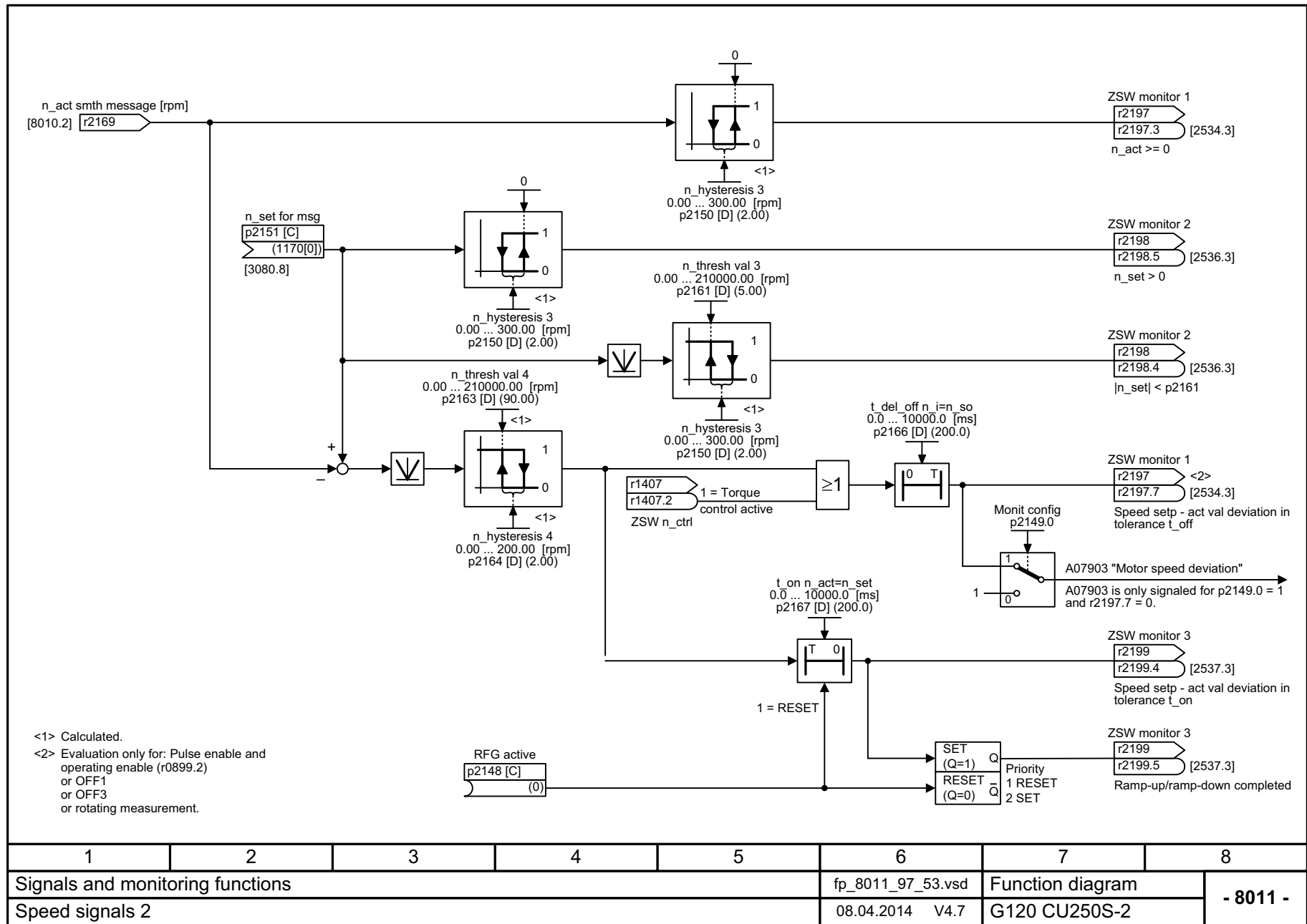
图 3-182 8011 - 转速信息 2
