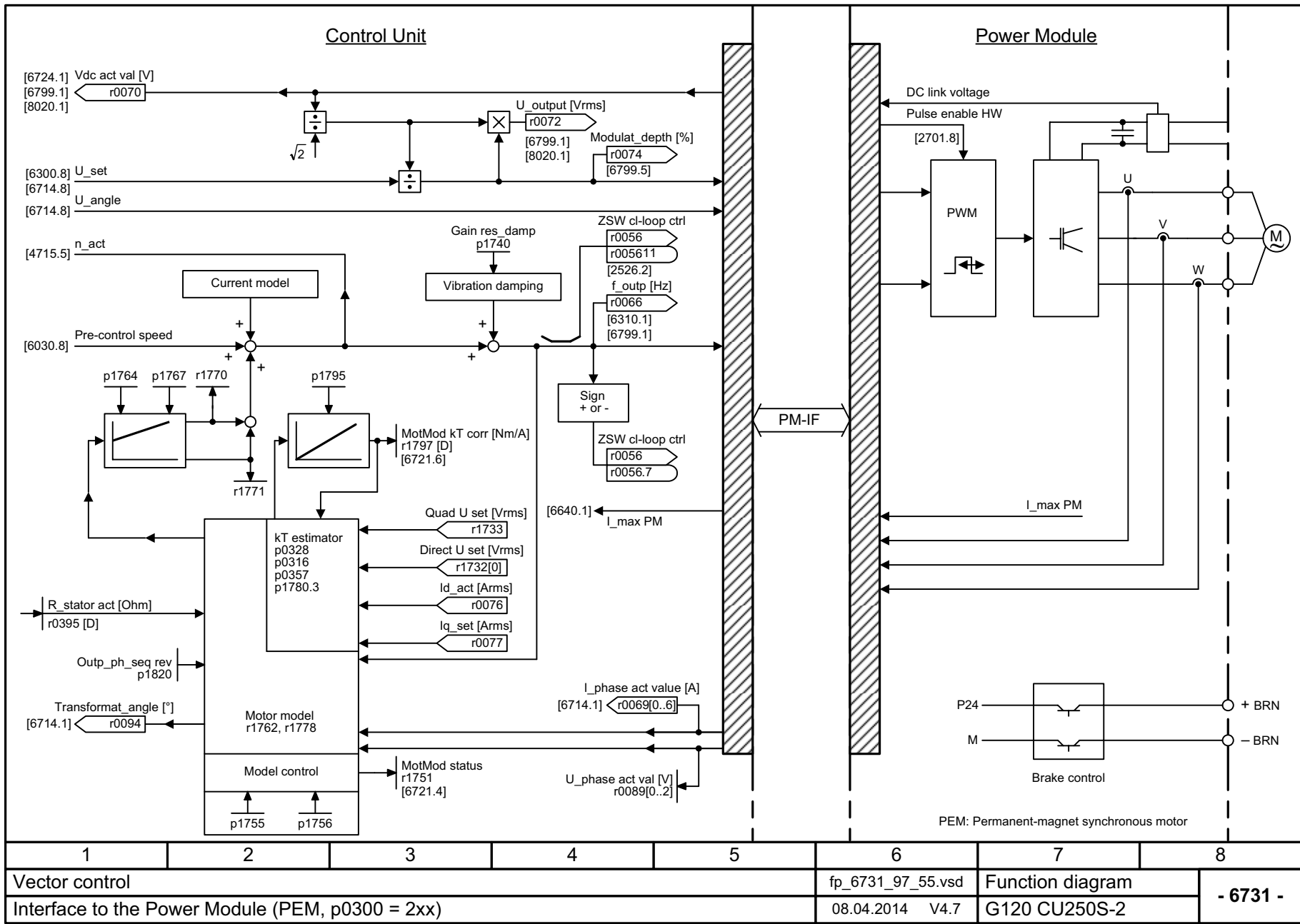
图 3-153 6731 - 和功率模块的接口 (PEM, p0300 = 2xx)
