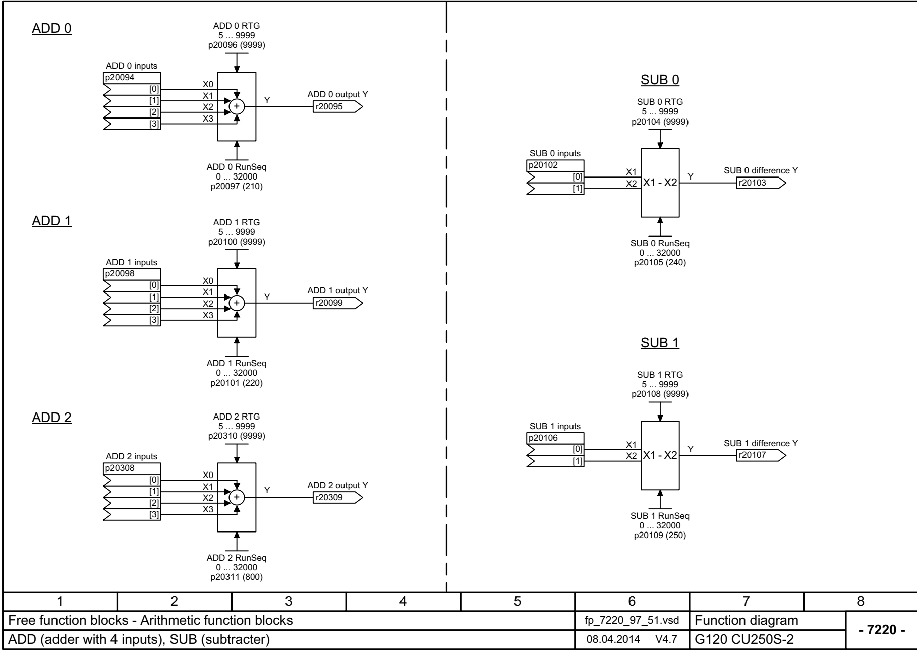
图 3-161 7220 - ADD (有 4 个输入的 加法器), SUB (减法器)
