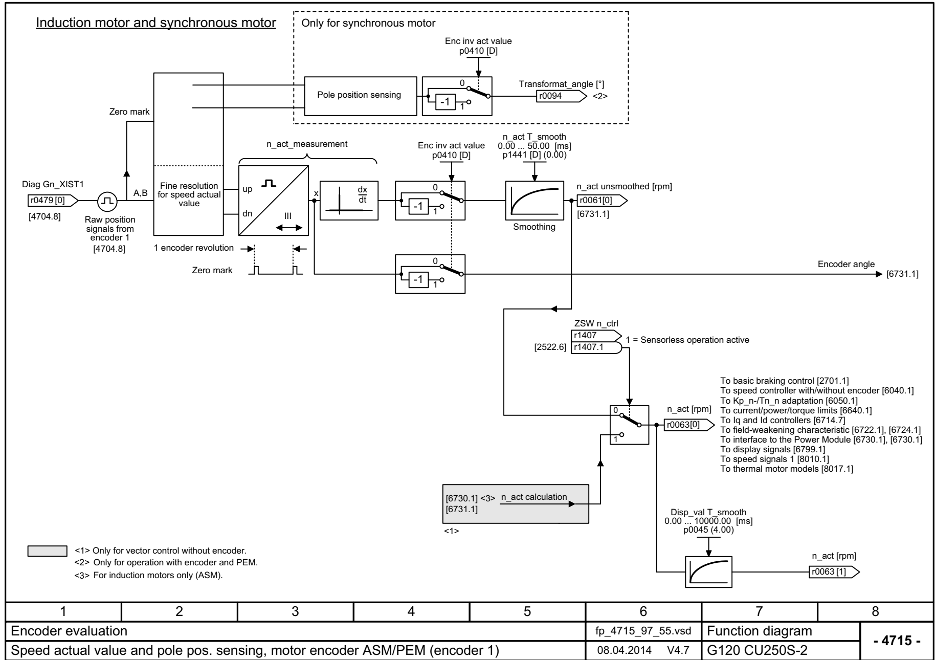
图 3-125 4715 - 转速实际值和极点位置采集电机编码器 ASM/SM (编码器 1)
