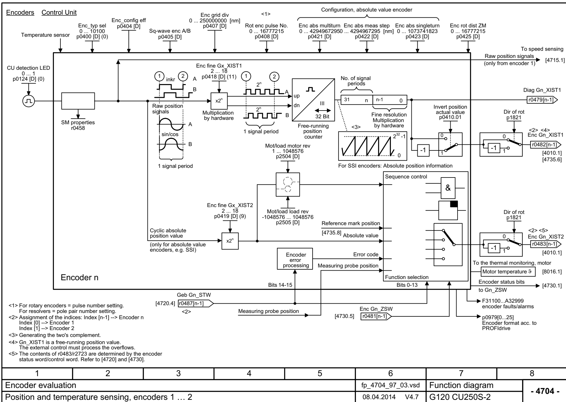
图 3-124 4704 - 位置和温度信号采集编码器 1 ... 2
