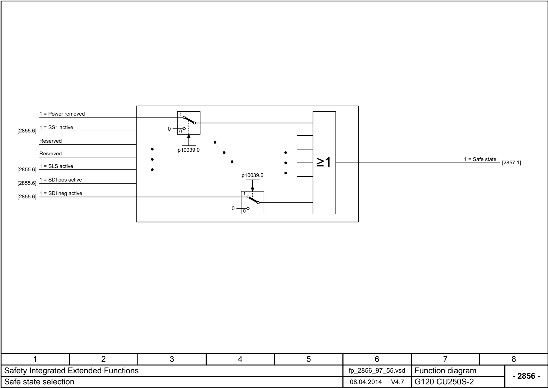
图 3-89 2856 - 安全状态选择
