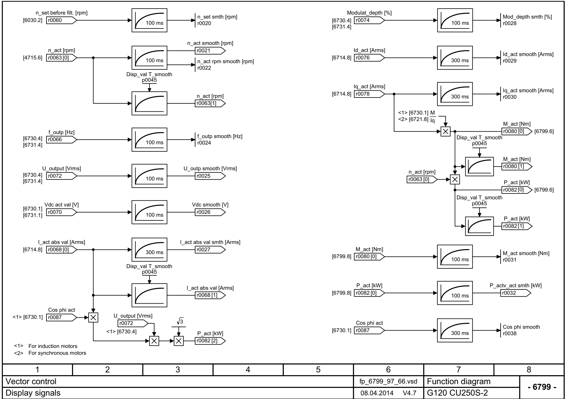
图 3-154 6799 - 显示信号
