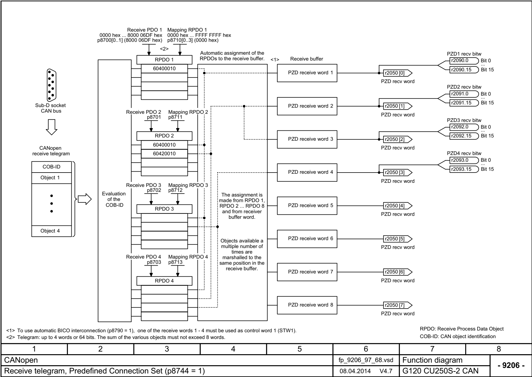
图 3-45 9206 - 预定义连接组接收报文 (p8744 = 1)
