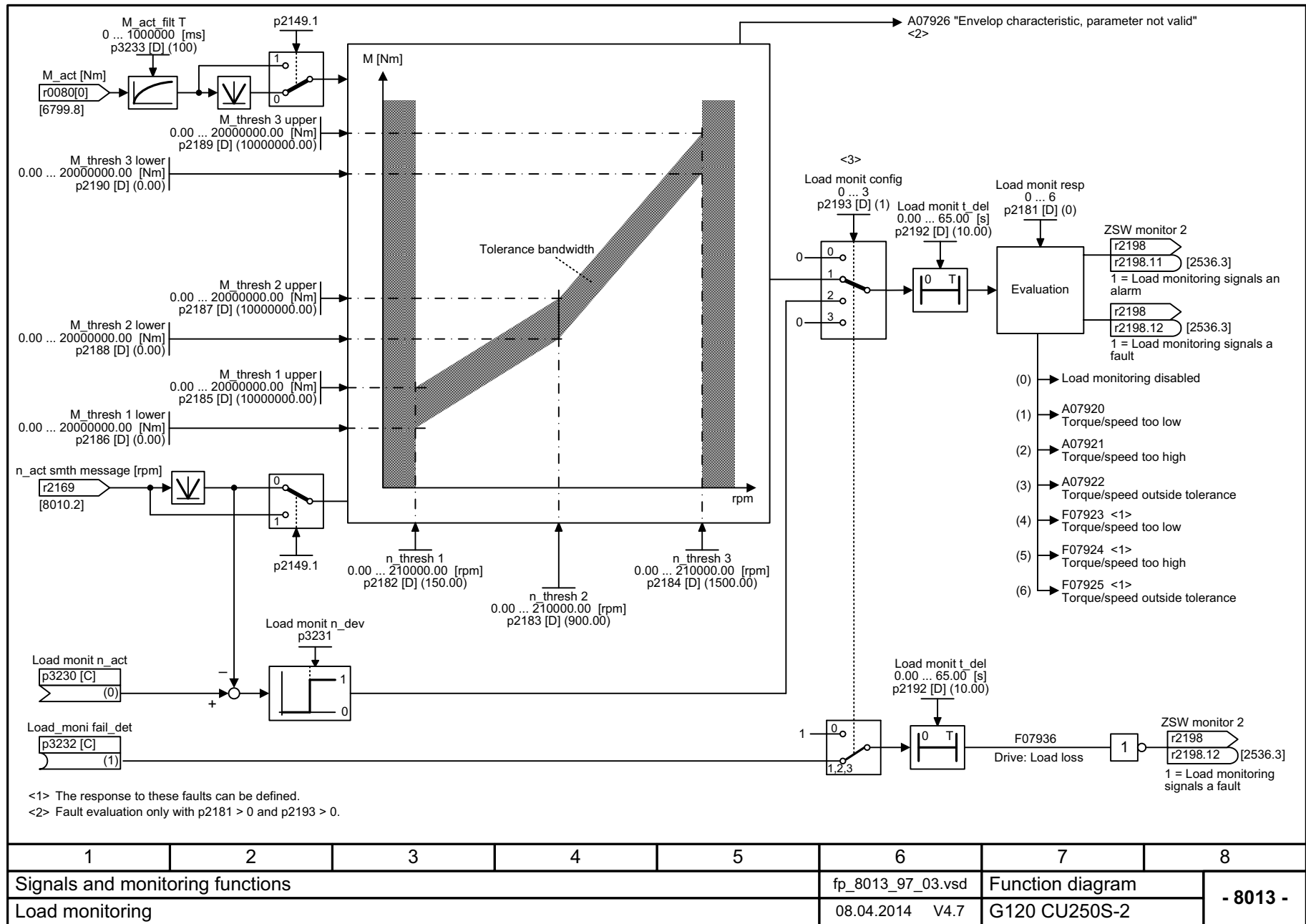
图 3-184 8013 - 负载监控
