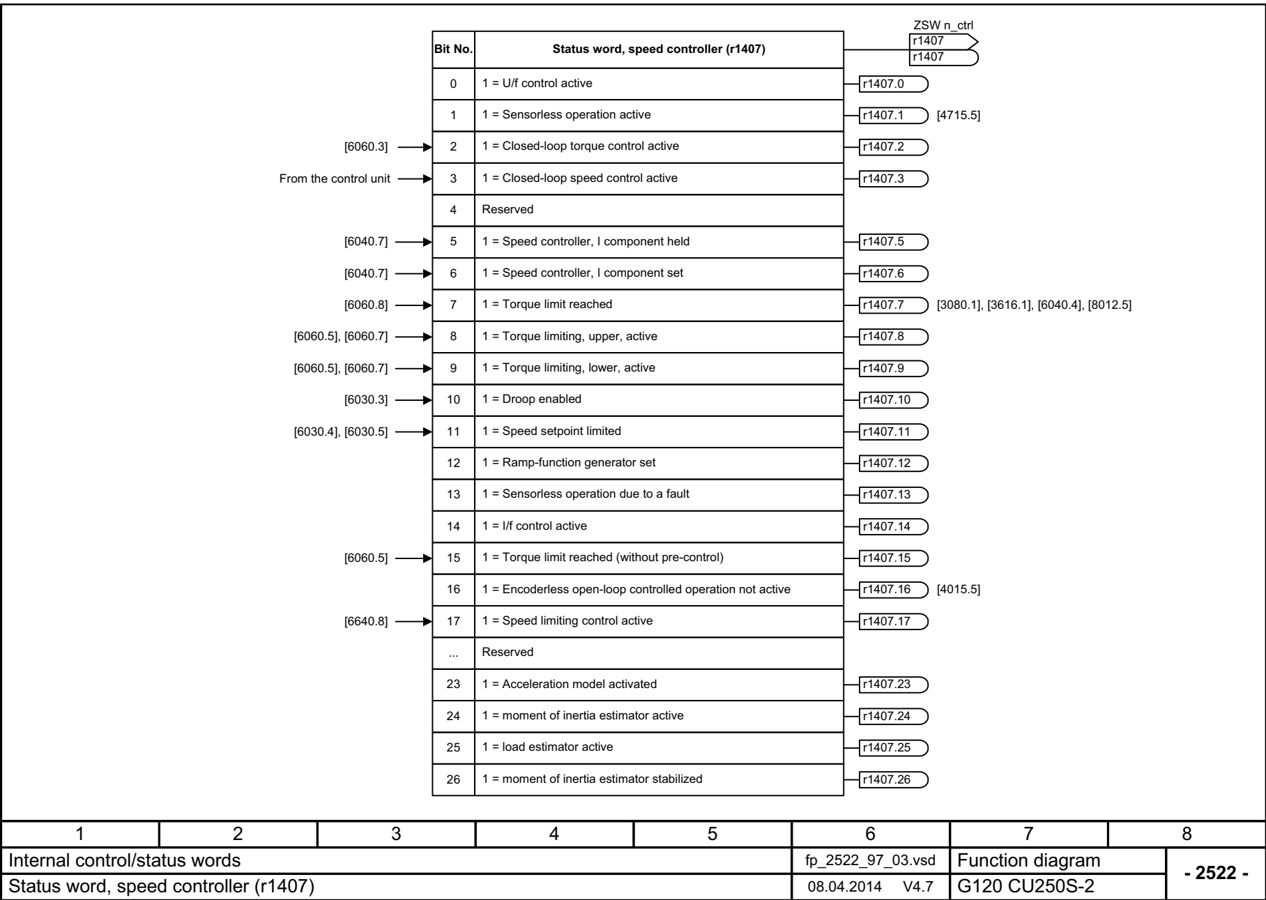
图 3-64 2522 - 转速控制器状态字 (r1407)
