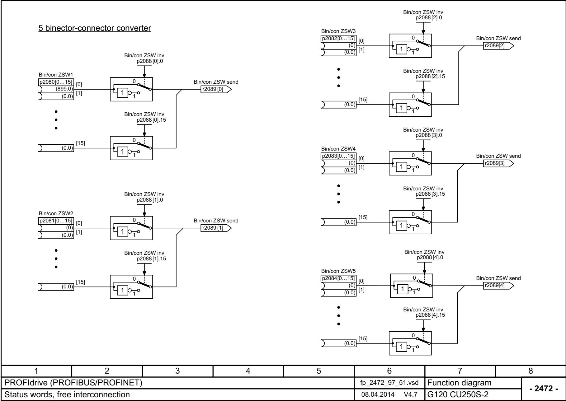
图 3-40 2472 - 自由互联状态字
