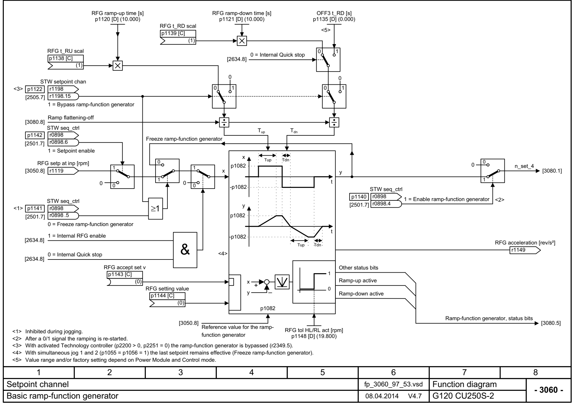
图 3-101 3060 - 简单斜坡函数发生器
