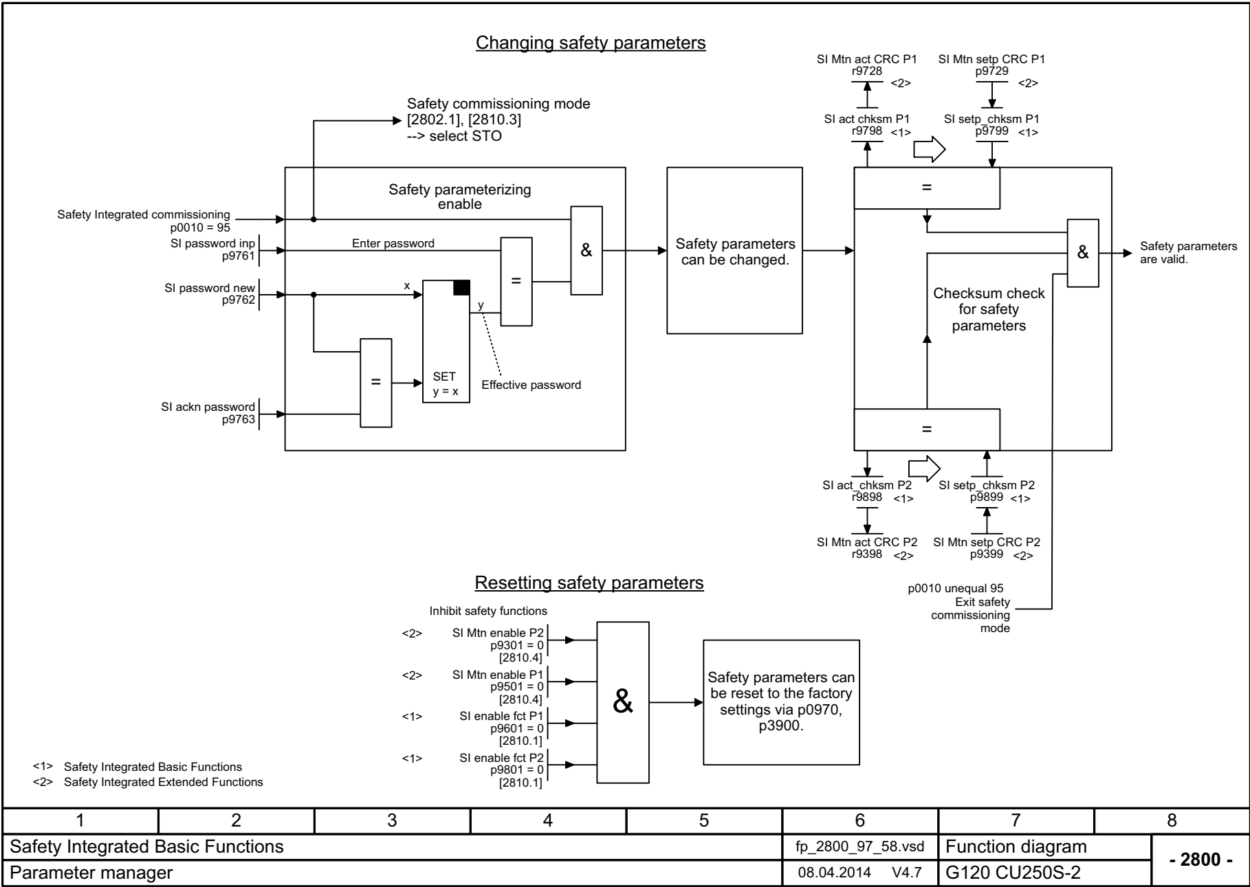
图 3-75 2800 - 参数管理器
