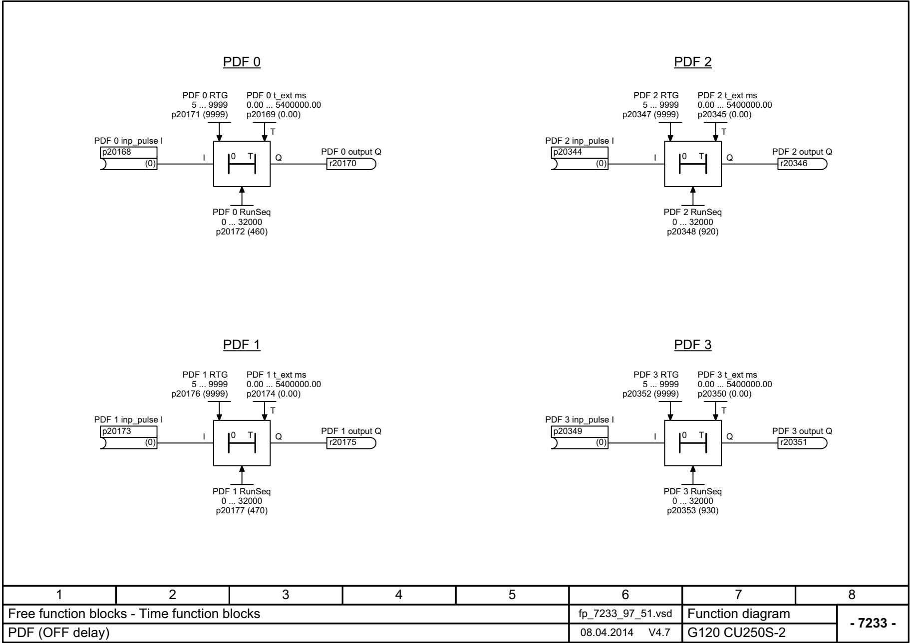
图 3-168 7233 - PDF (关闭延迟)
