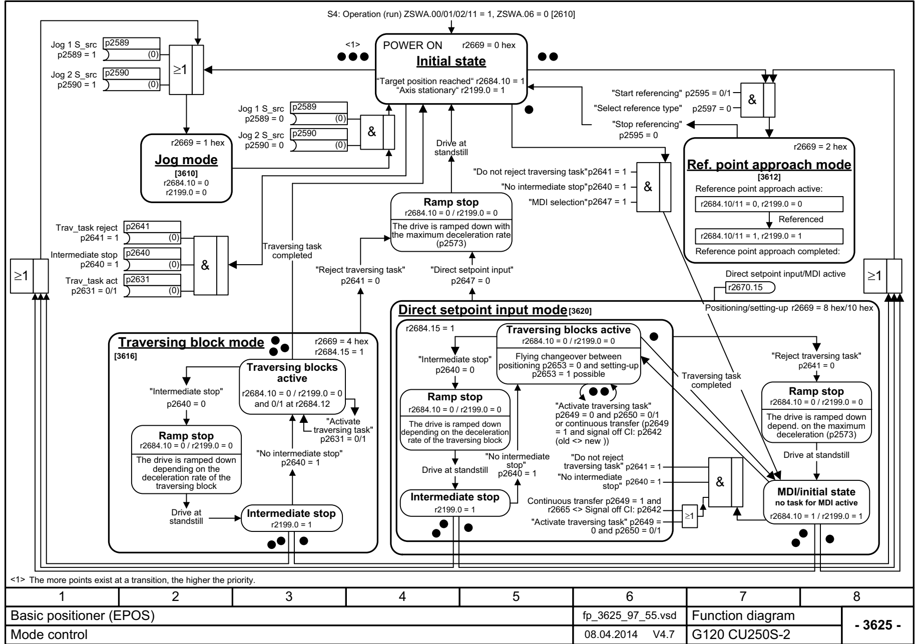
图 3-113 3625 - 运行方式控制
