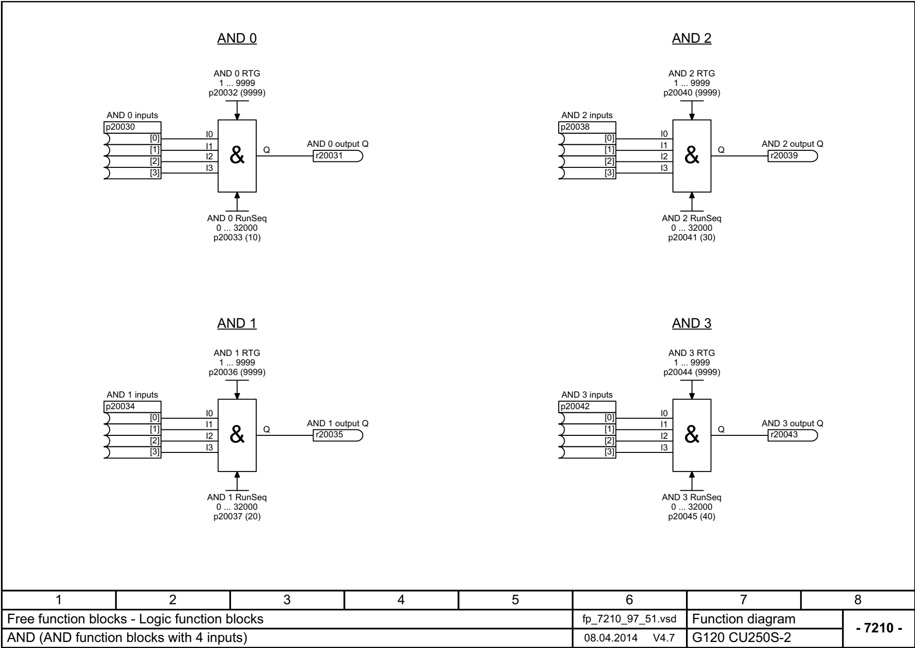
图 3-157 7210 - AND (有 4 个输入的 “与” 功能块)
