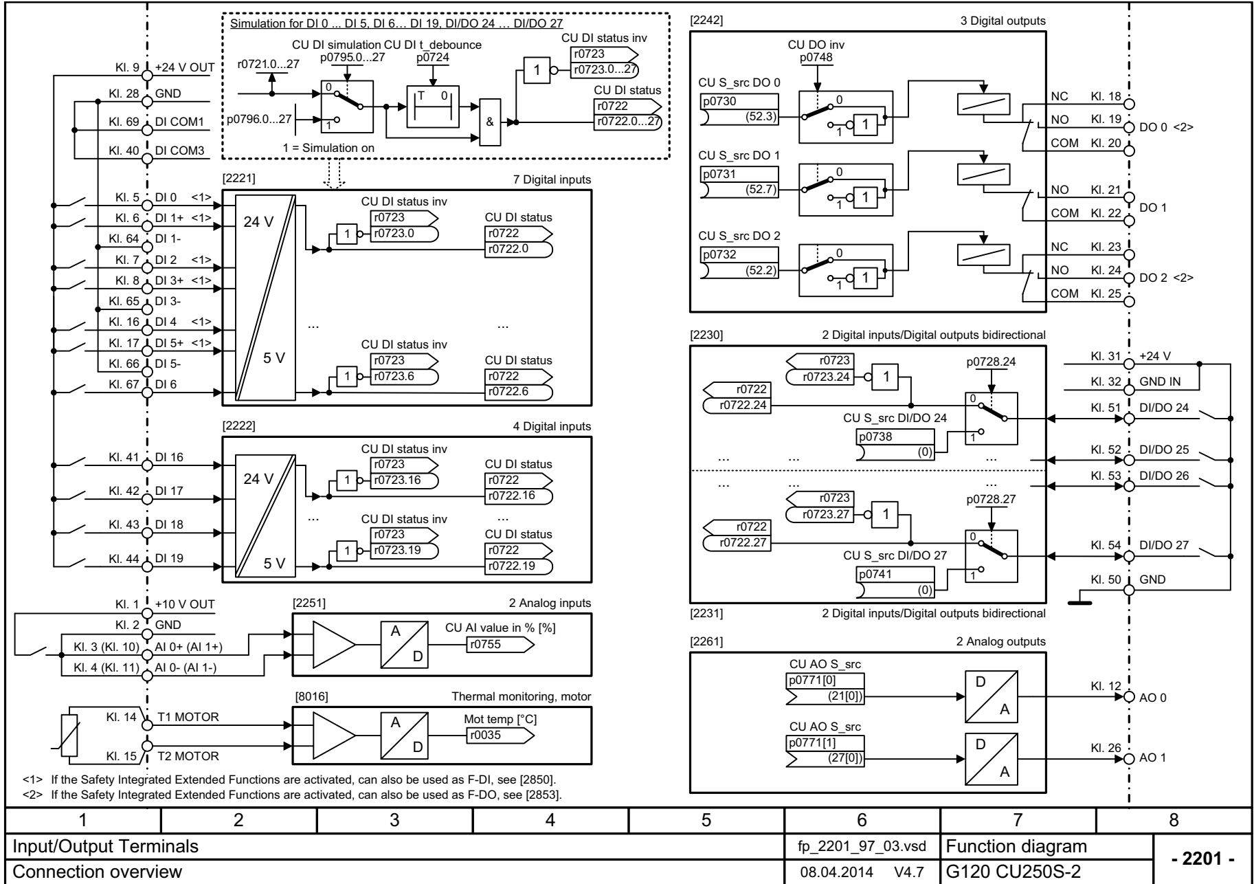
图 3-5 2201 - 接口一览
