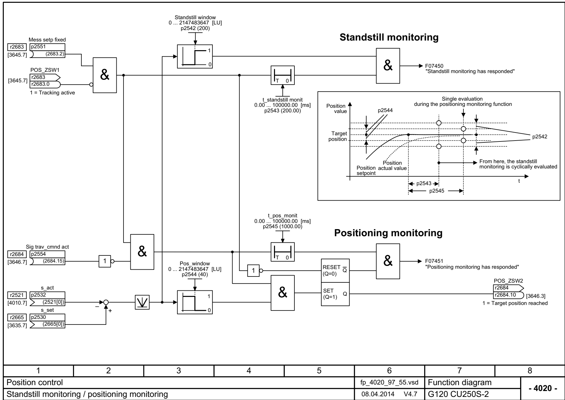
图 3-122 4020 - 静态监控 / 定位监控
