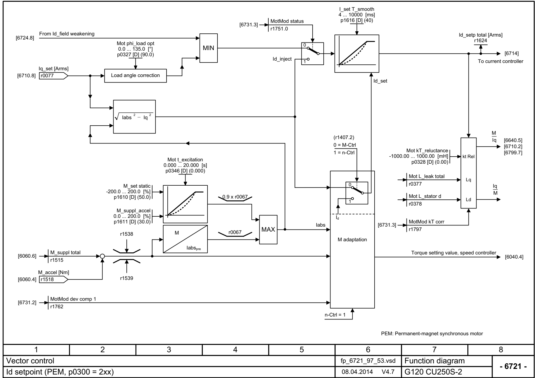
图 3-148 6721 - Id 设定值 (PEM, p0300 = 2xx)
