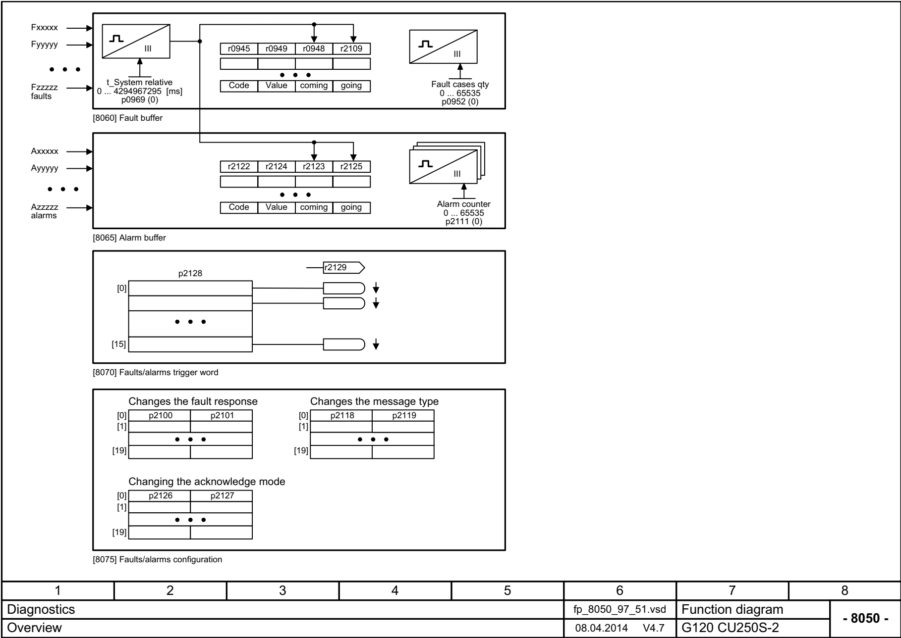
图 3-190 8050 - 一览
