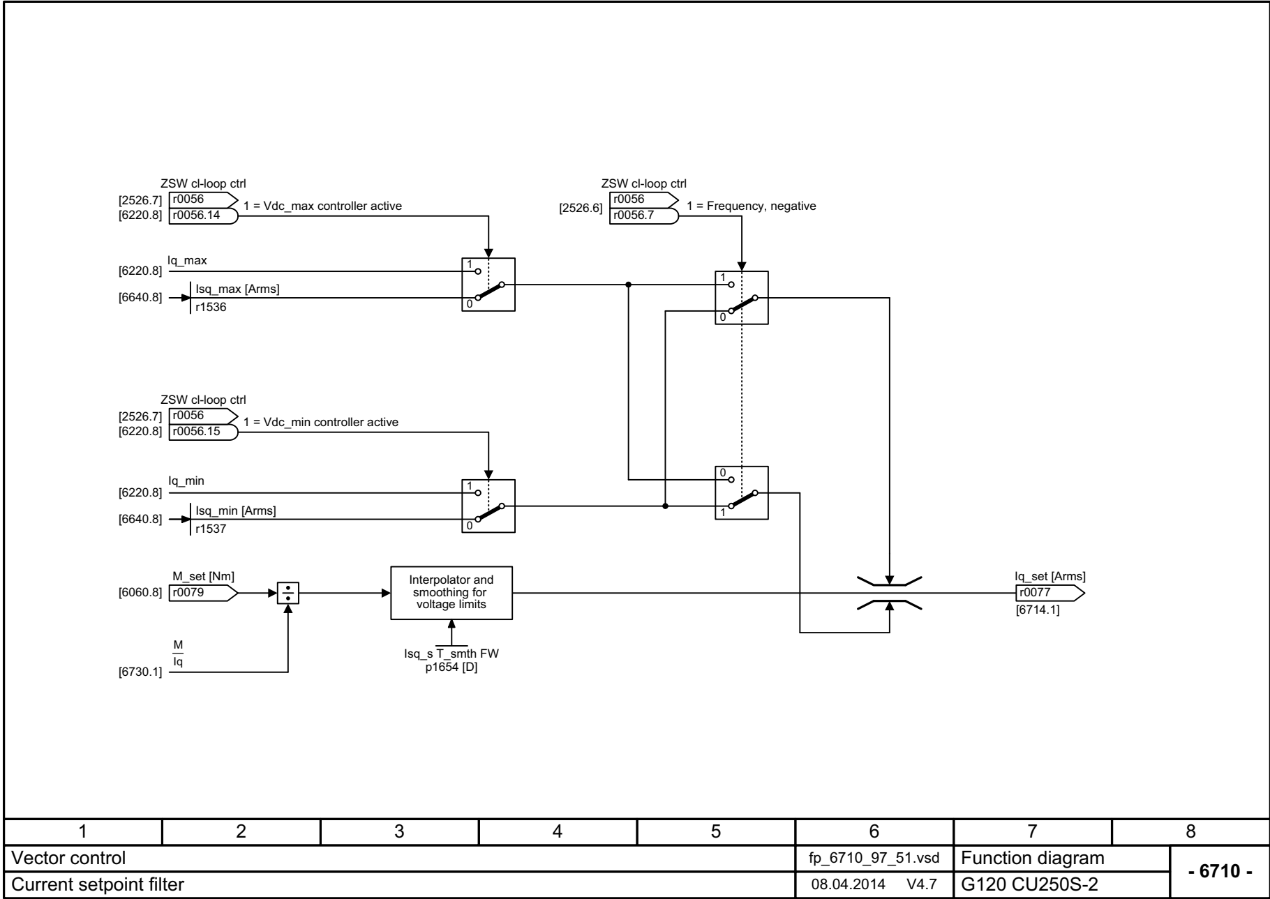
图 3-146 6710 - 电设定值滤波器
