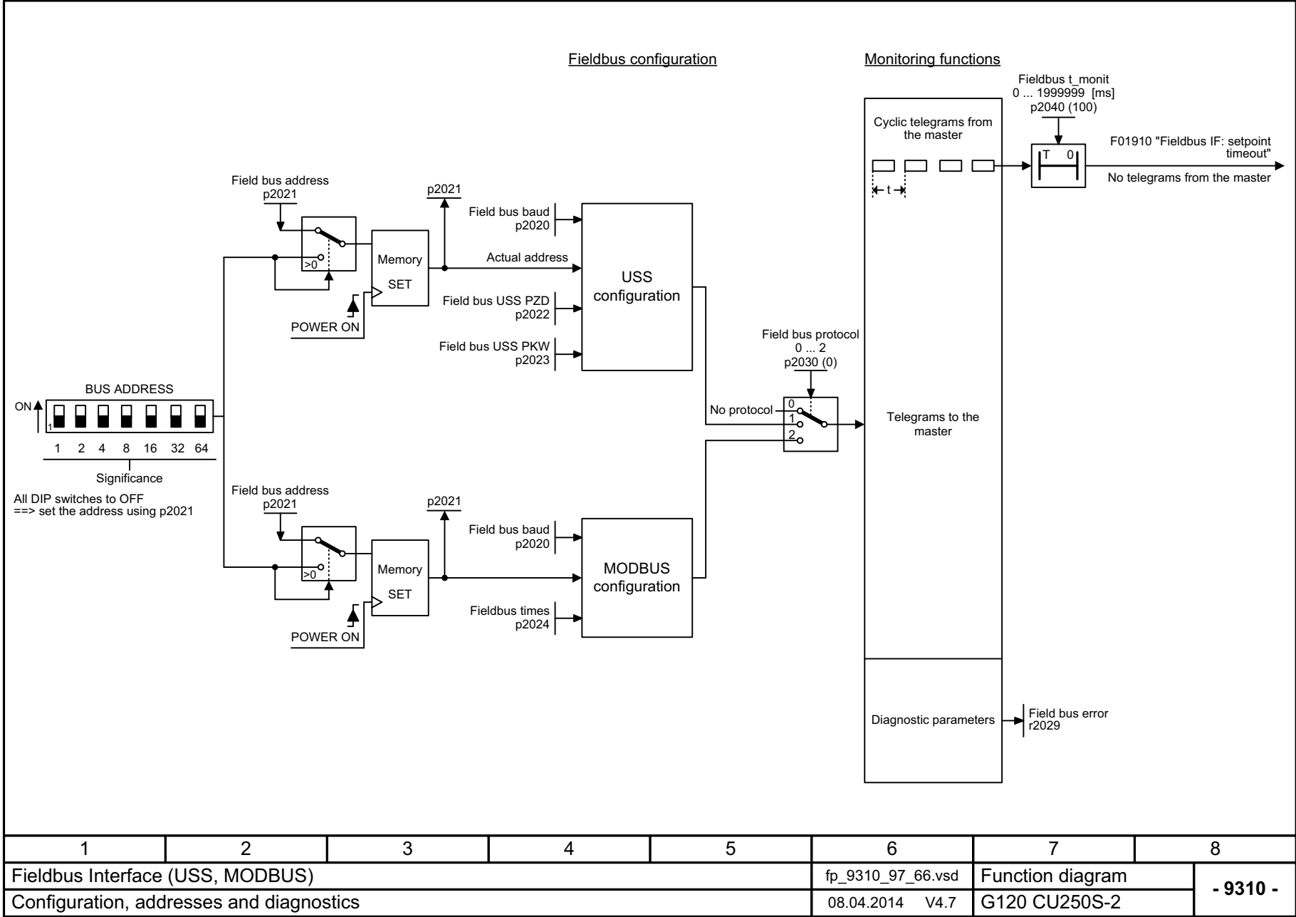
图 3-50 9310 - 配置，地址及诊断
