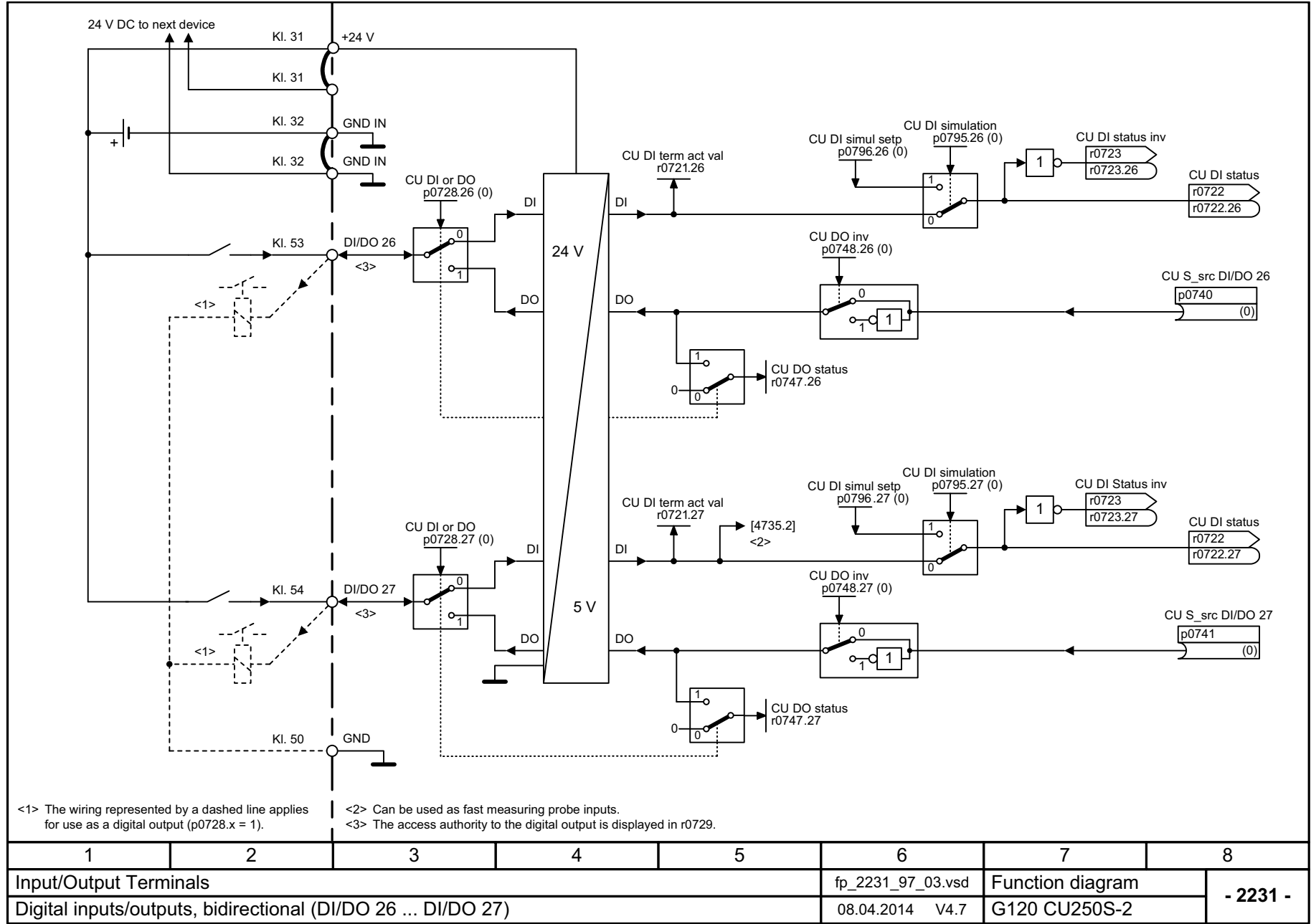
图 3-9 2231 - 双向数字输入端 / 输出端 (DI/DIO 26 ... DI/DO 27)
