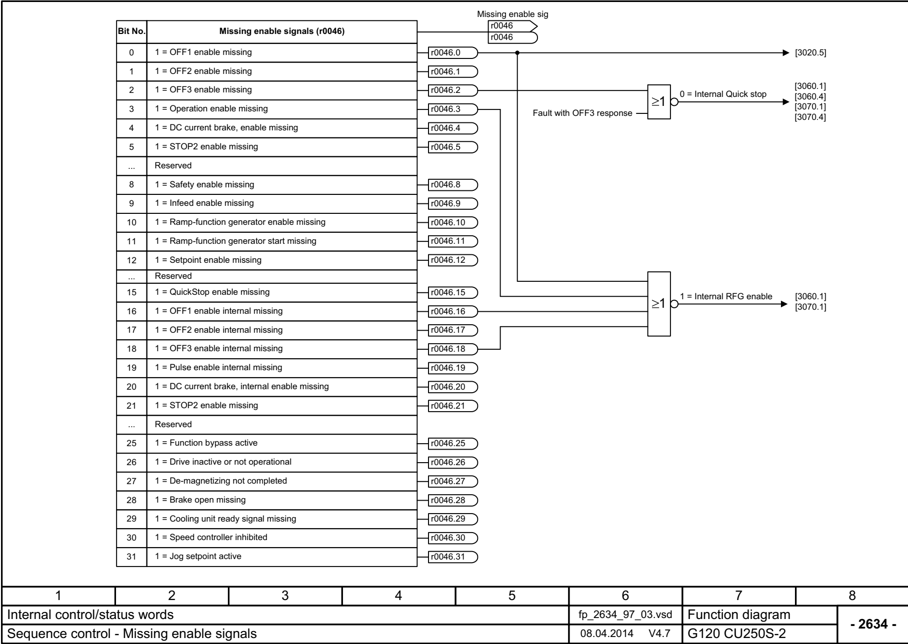
图 3-73 2634 - 顺序控制 - 缺少使能信号 (矢量控制)
