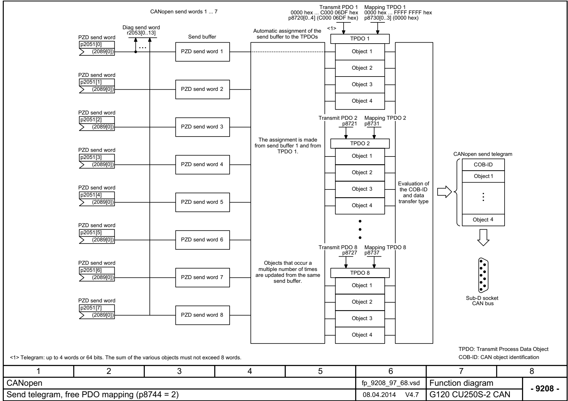
图 3-46 9208 - 由 PDO 映射发送报文 (p8744 = 2)
