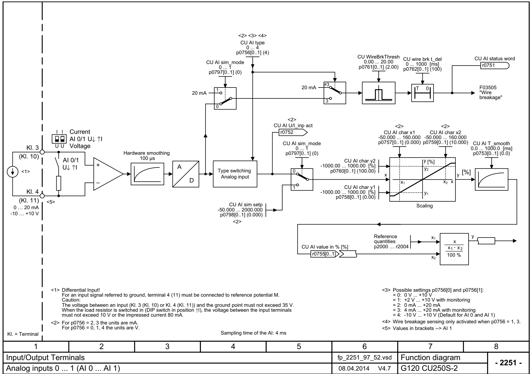
图 3-11 2251 - 模拟输入端 0 ... 1 (AI 0 ... AI 1)
