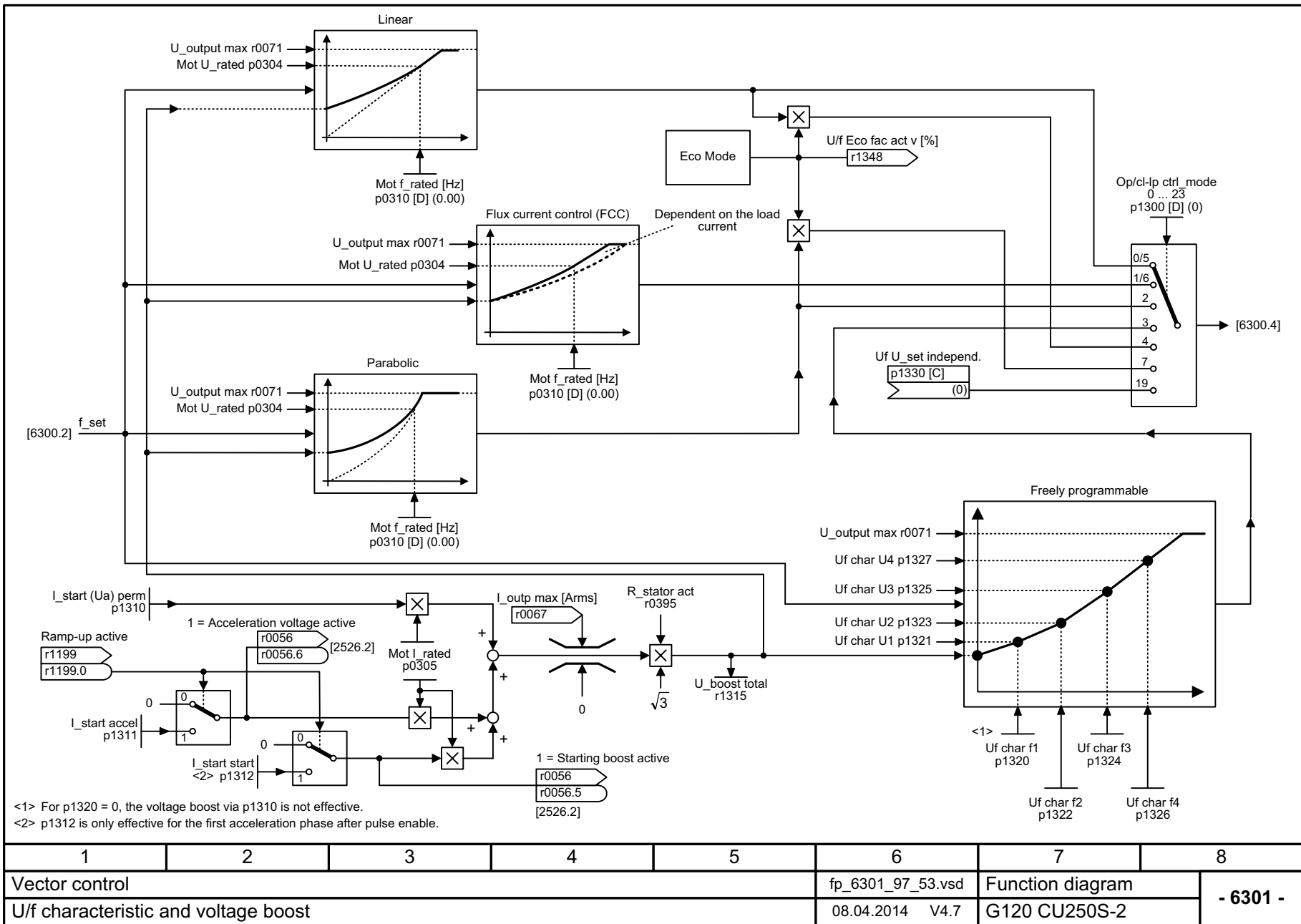
图 3-138 6301 - V/f 特性曲线和压升
